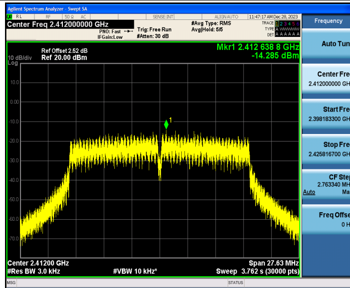
802.11n(HT20)_Ant2_2412
