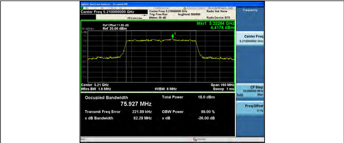
11AC80MIMO_Ant2_5210
