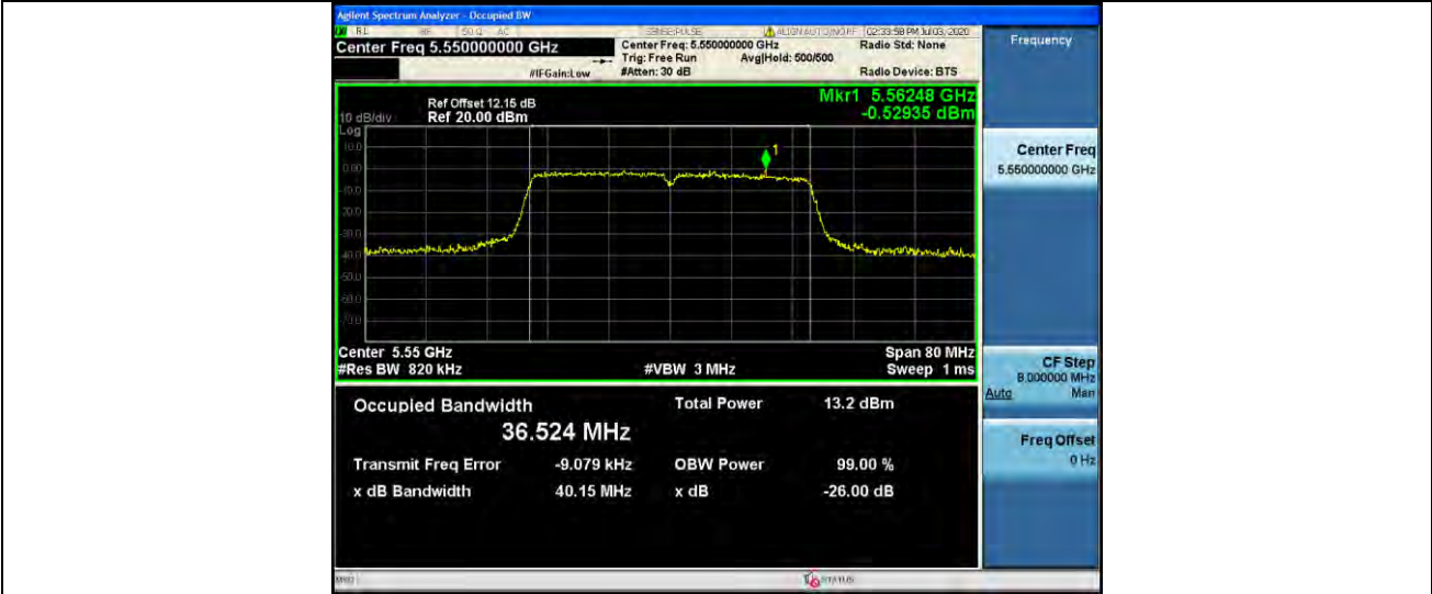
11N40MIMO_Ant2_5550
