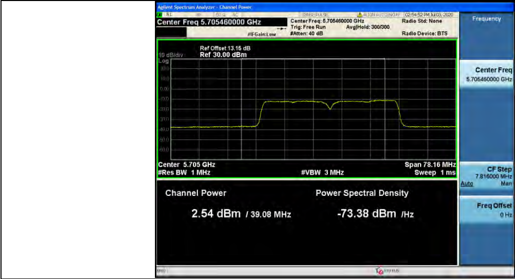
11N40MIMO_Ant1_5710_UNII-3
