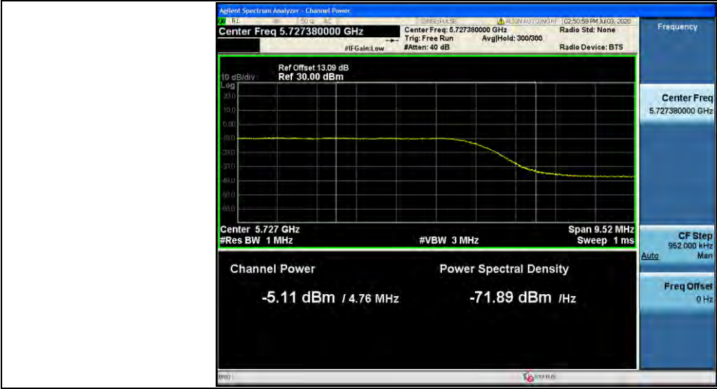
11N40MIMO_Ant2_5710_UNII-3
