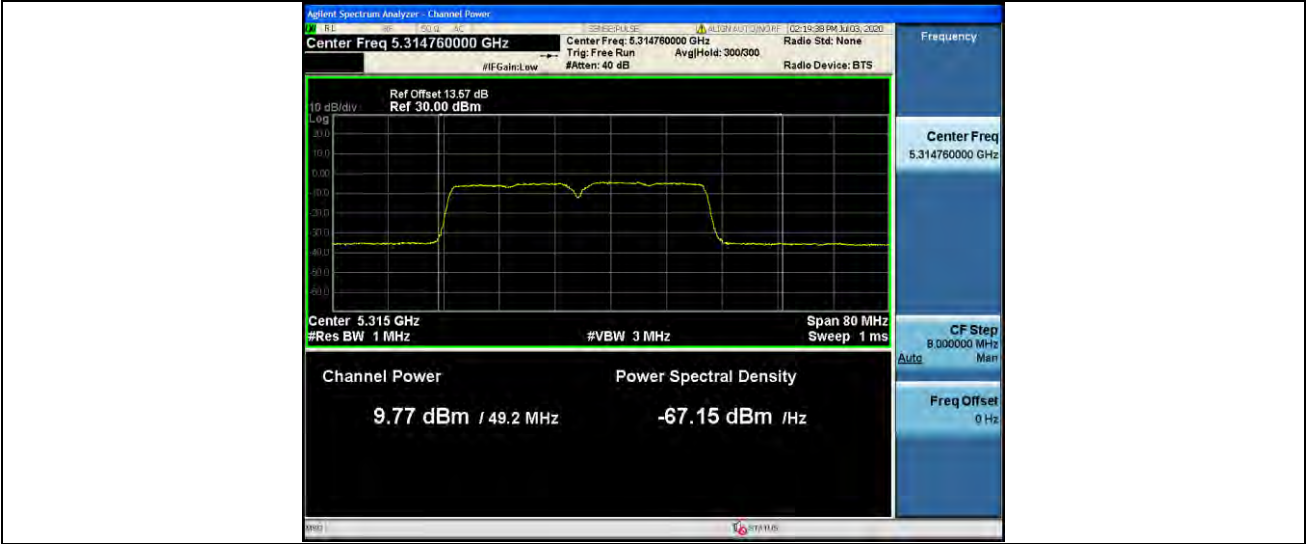
11N40MIMO_Ant2_5310
