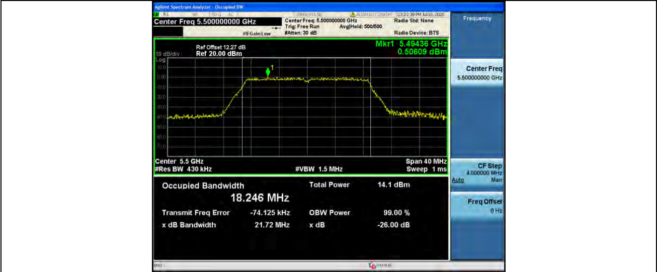
11AC20MIMO_Ant2_5500
