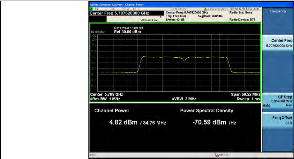
11N40MIMO_Ant2_5710_UNII-2C
