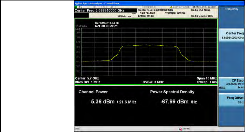
11A_Ant2_5700
