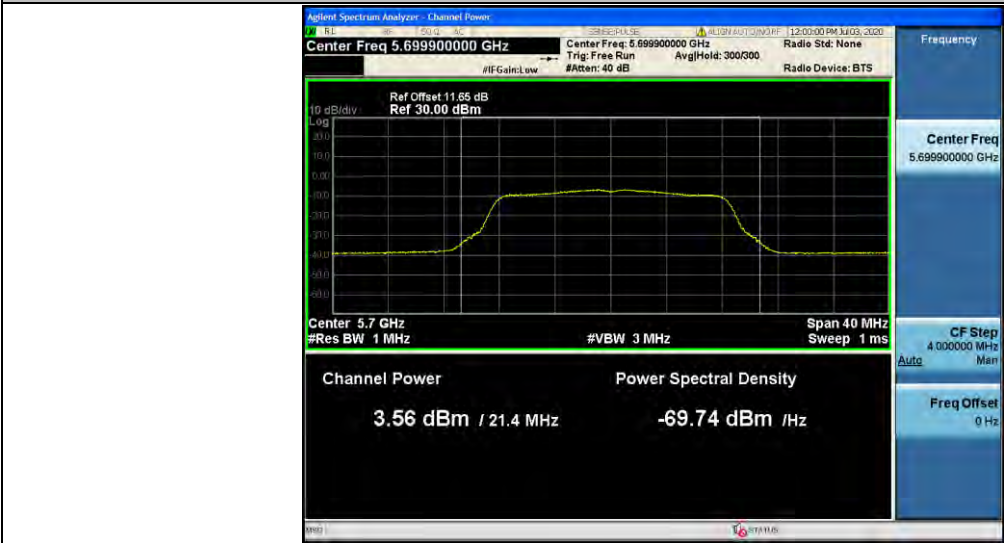
11A_Ant1_5720_UNII-2C
