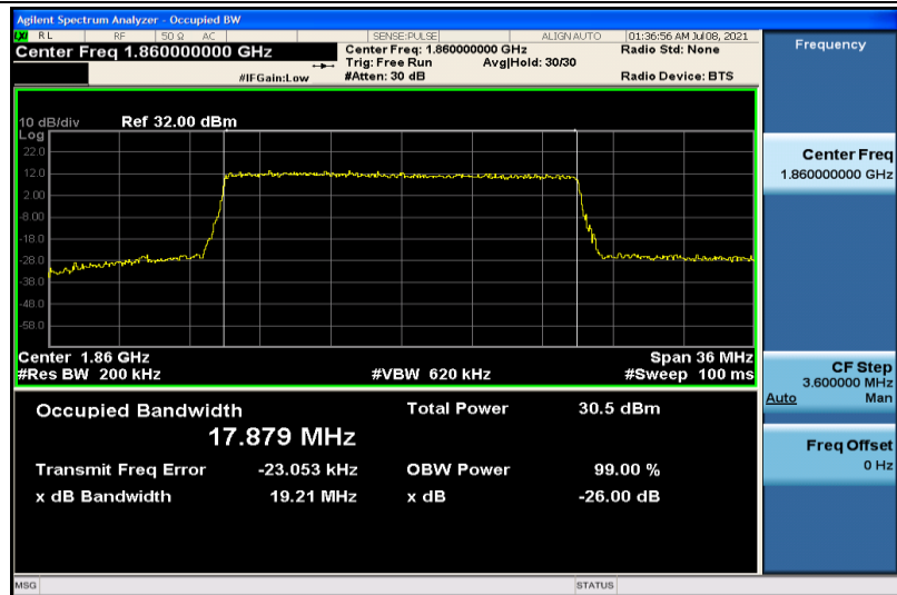
Band2-20MHz-QPSK-18700-100RB#0-17.879
