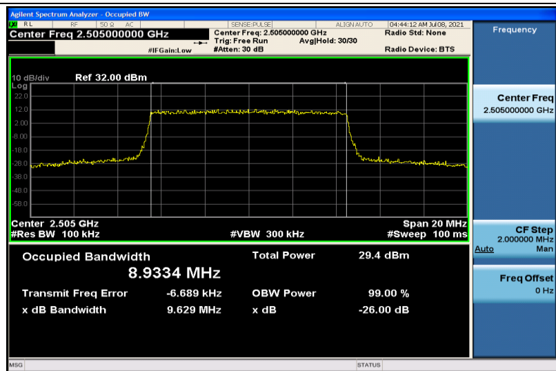
Band7-10MHz-QPSK-20800-50RB#0-8.9334
