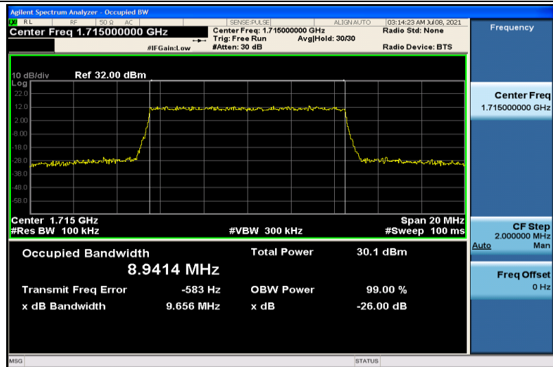
Band4-10MHz-QPSK-20000-50RB#0-8.9414
