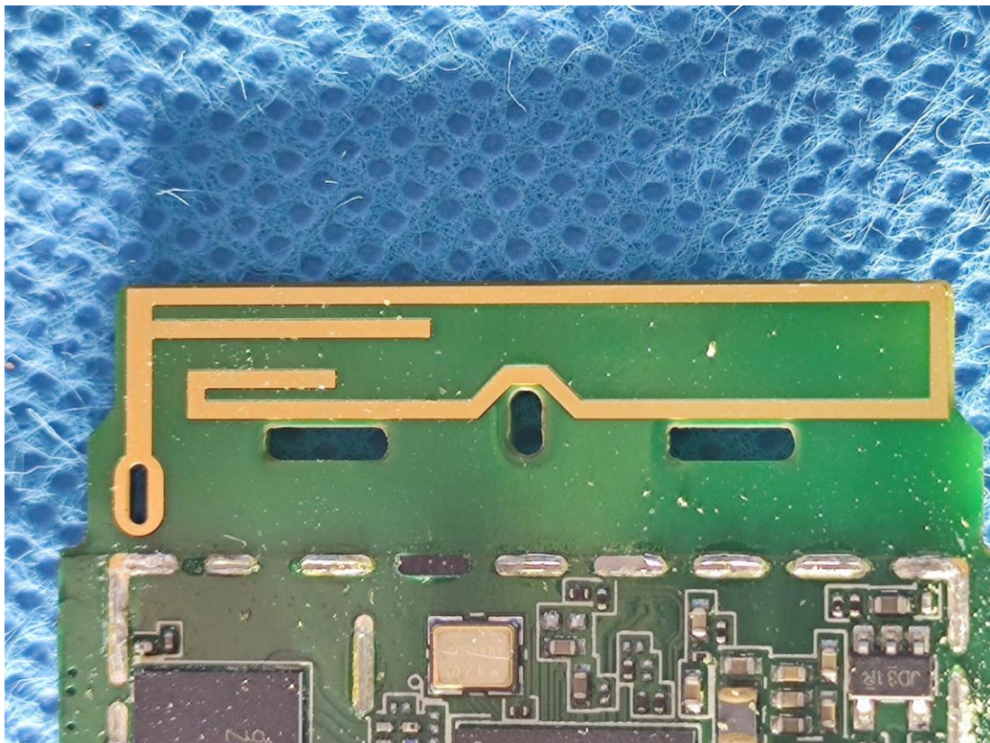
GSM Antenna
