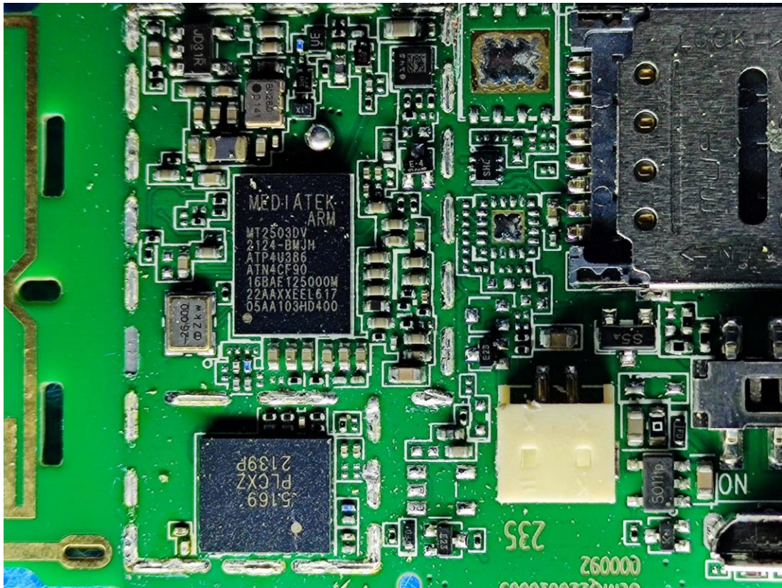
GSM Antenna
