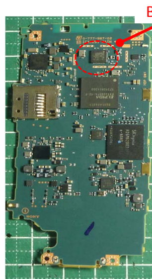
PWB IC side
