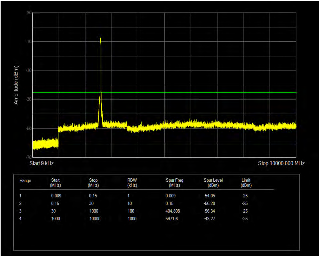
n41 SCS=30kHz CP_QPSK BW=40MHz Channel=518598 RB=1@0
