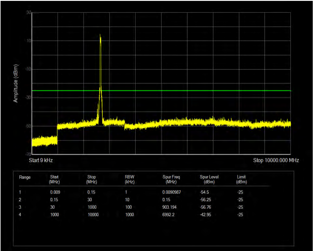
n41 SCS=30kHz CP_QPSK BW=40MHz Channel=534000 RB=1@0
