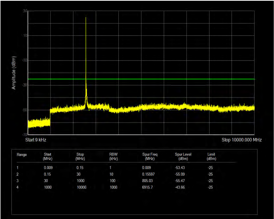
n41 SCS=30kHz CP_QPSK BW=40MHz Channel=518598 RB=1@105
