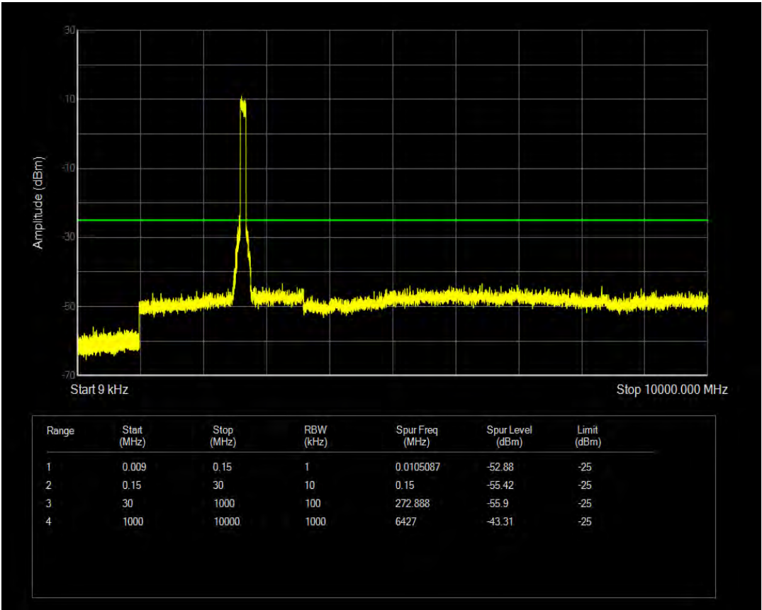
n41 SCS=30kHz CP_QPSK BW=90MHz Channel=528996 RB=1@0
