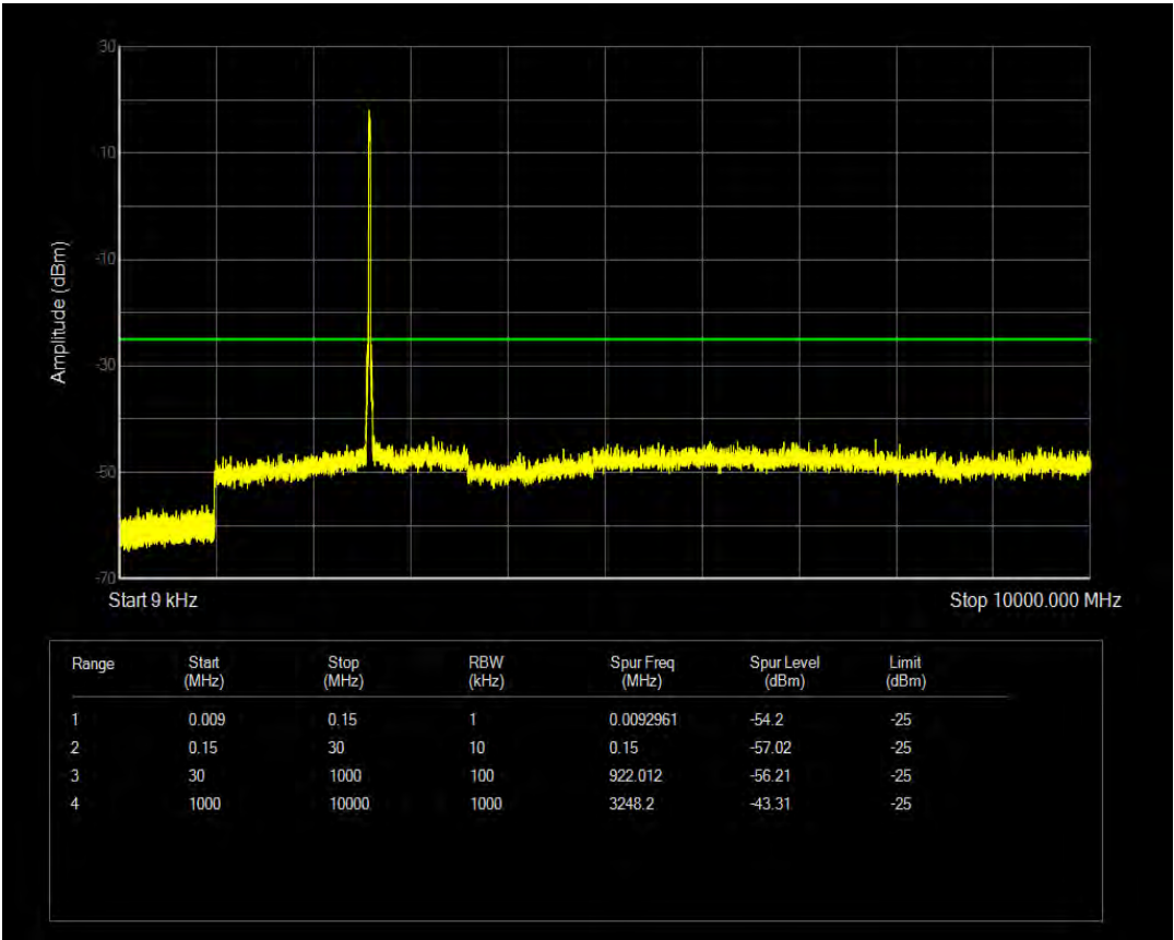
n41 SCS=30kHz CP_QPSK BW=20MHz Channel=518598 RB=1@0
