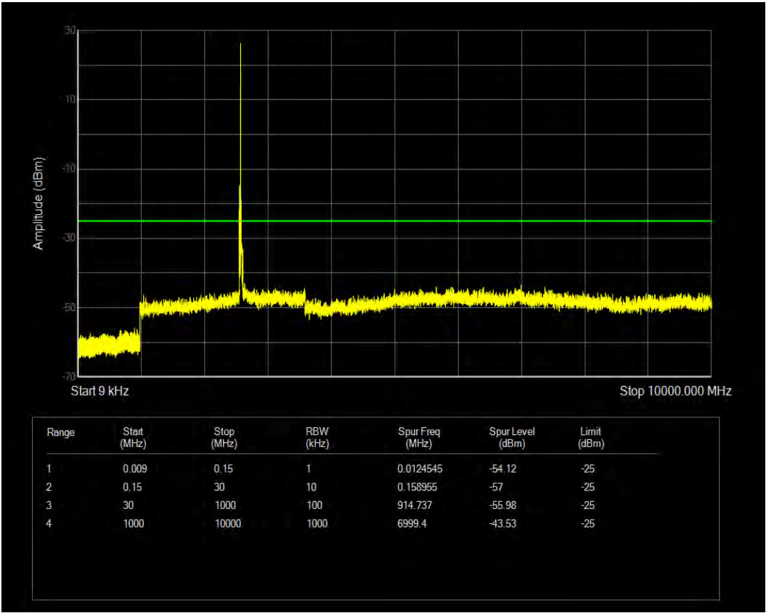
n41 SCS=30kHz CP_QPSK BW=20MHz Channel=518598 RB=1@50
