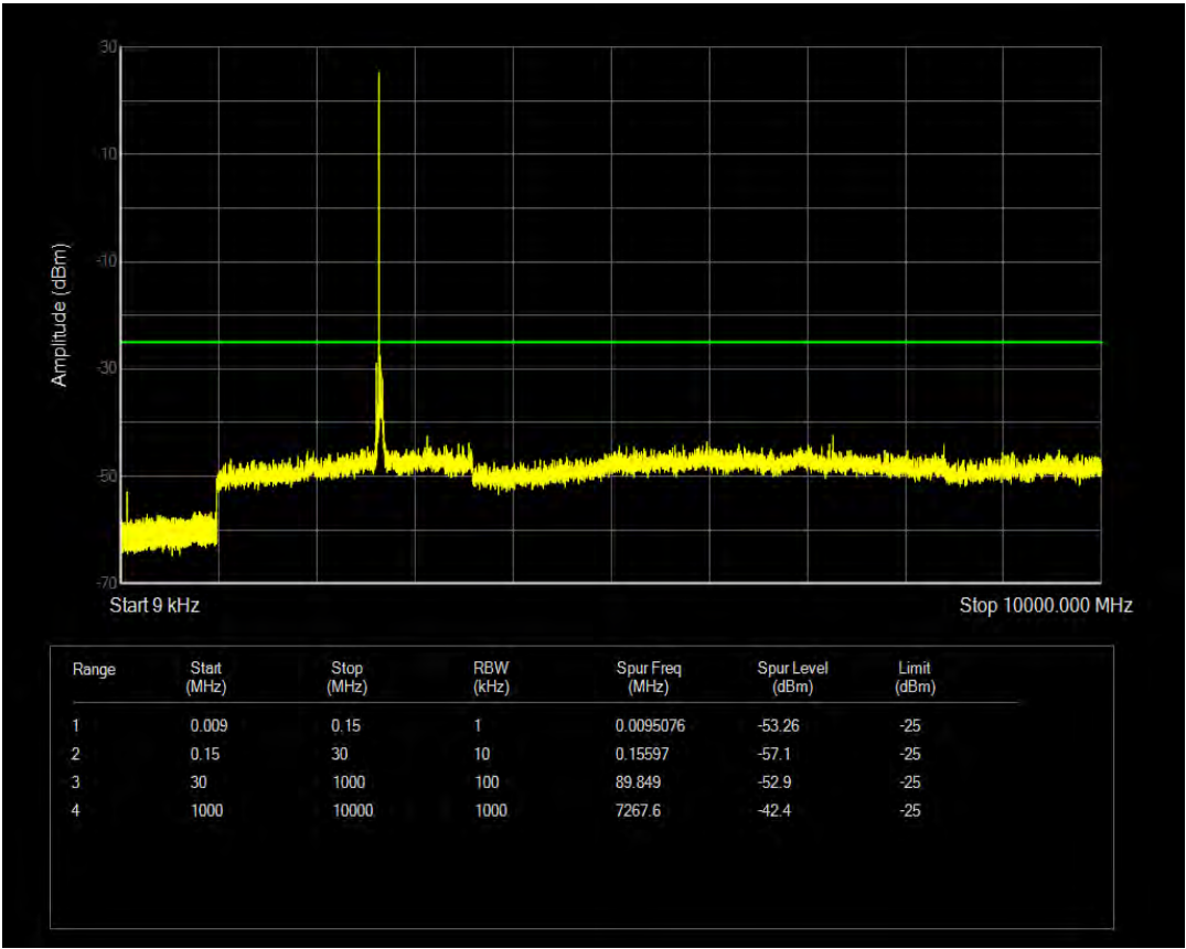
n41 SCS=30kHz CP_QPSK BW=40MHz Channel=534000 RB=1@105
