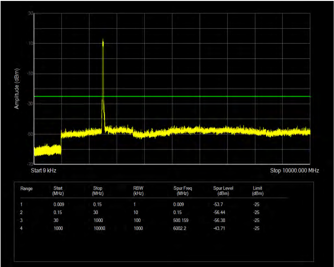
n41 SCS=30kHz CP_QPSK BW=40MHz Channel=503202 RB=1@0
