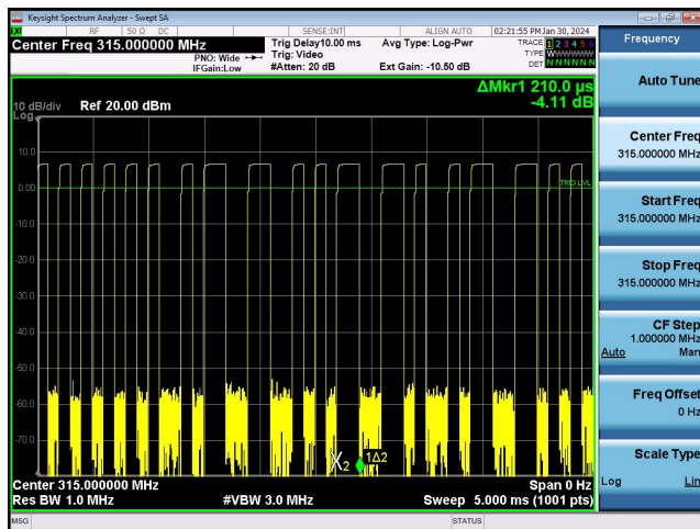
315 MHz: Burst 1
