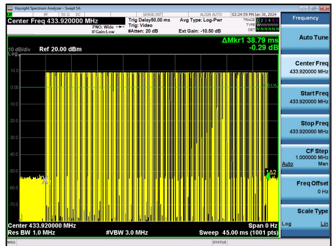
433.92 MHz: Burst 2
