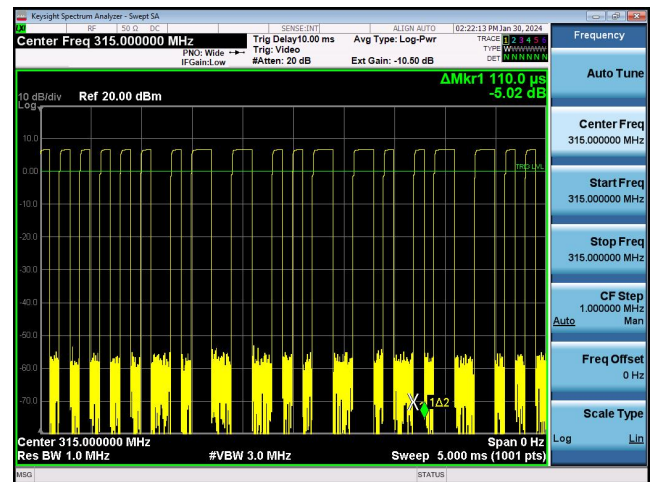
315 MHz: Burst 2
