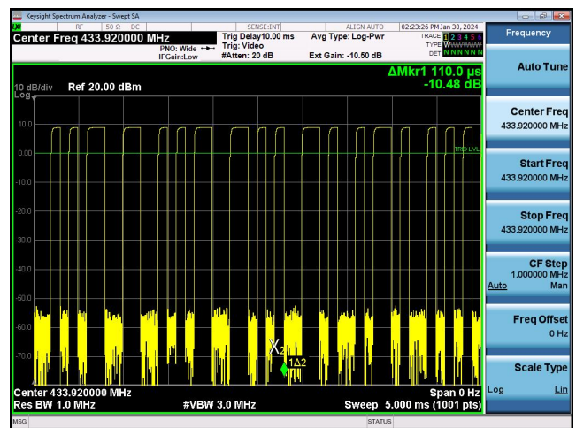
433.92 MHz: Burst 2
