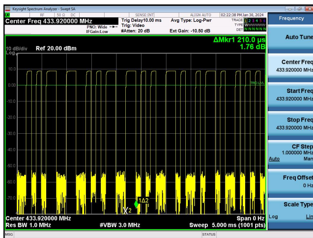
433.92 MHz: Burst 1
