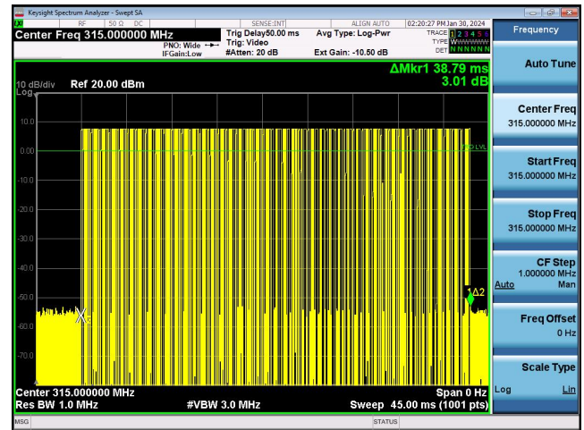
315 MHz: Burst 2
