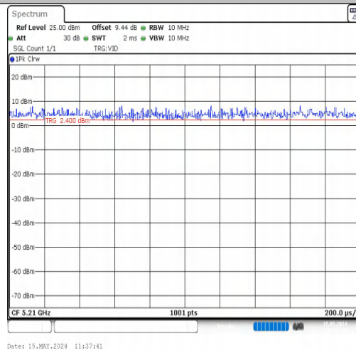
NTNV-11AC80MIMO-Ant1-5210
