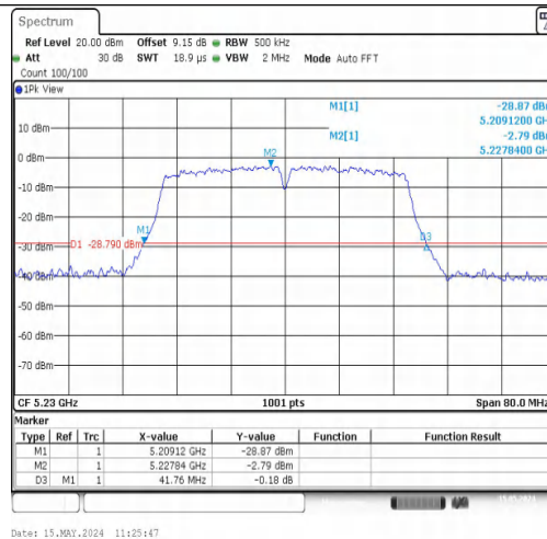
11N40MIMO-Ant2-5230
