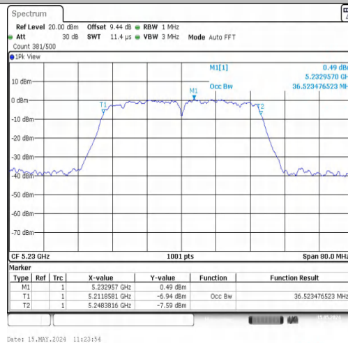
11N40MIMO-Ant1-5230
