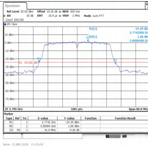
11N40MIMO-Ant1-5795
