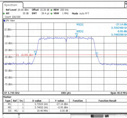
11N20MIMO-Ant1-5745
