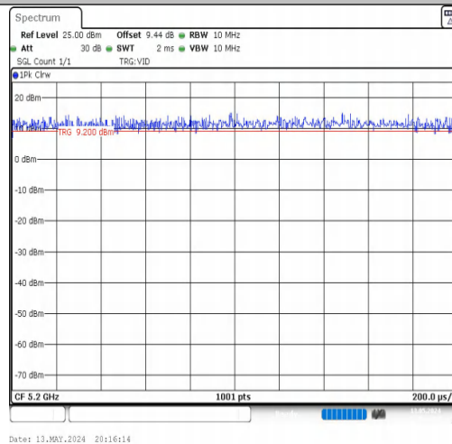
NTVN-11N20MIMO-Ant1-5200
