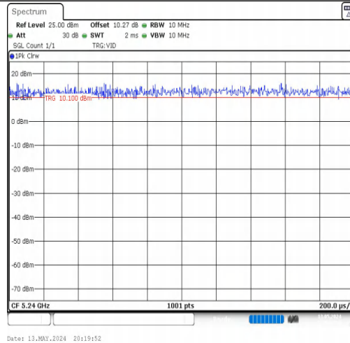
NTNV-11N20MIMO-Ant1-5240
