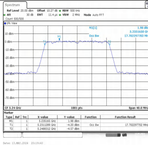
11N20MIMO-Ant1-5240
