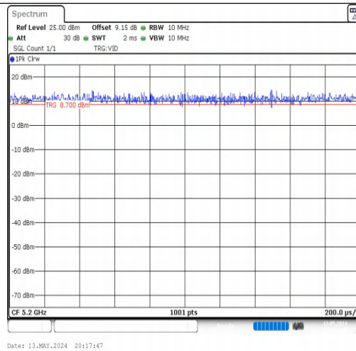
NTNV-11N20MIMO-Ant2-5200
