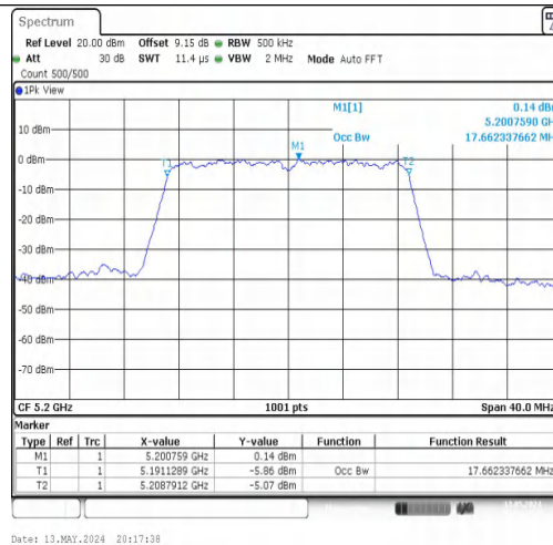
11N20MIMO-Ant2-5200
