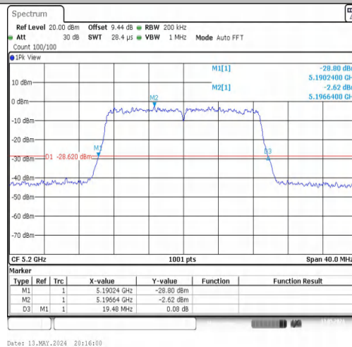
11N20MIMO-Ant1-5200
