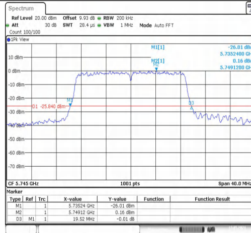
11N20MIMO-Ant1-5745
