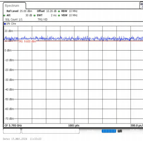
NTNV-11N40MIMO-Ant1-5795
