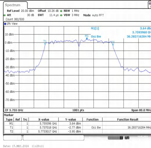
11N40MIMO-Ant1-5755
