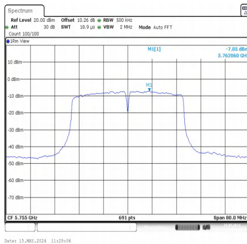
11N40MIMO-Ant1-5755-PASS
