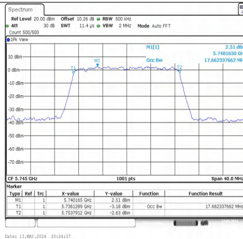
11N20MIMO-Ant1-5745
