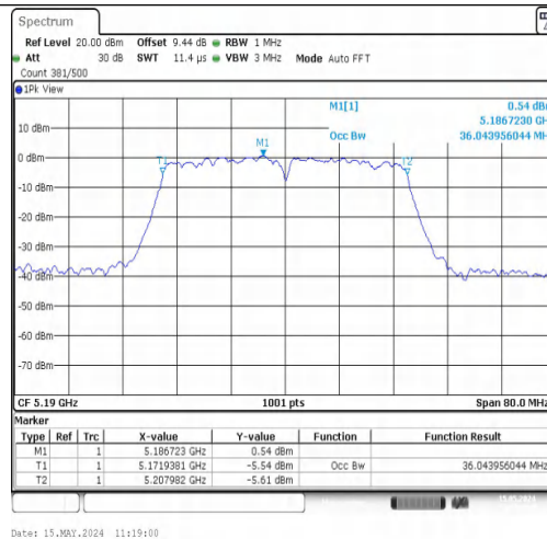
11N40MIMO-Ant1-5190
