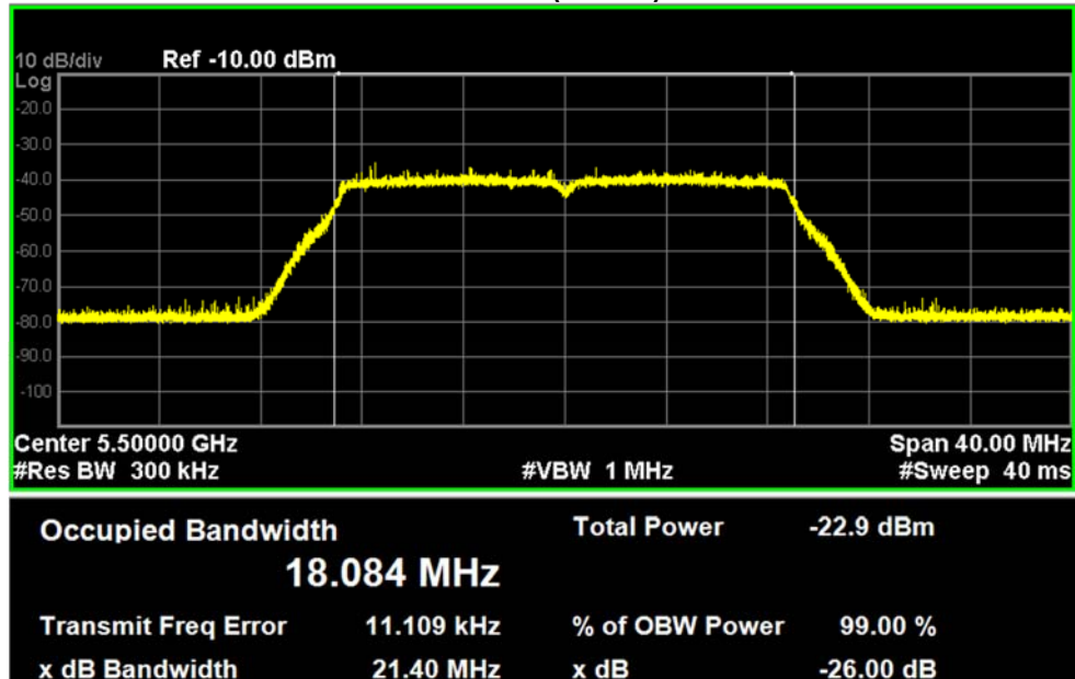
802.11ac (VHT20)
