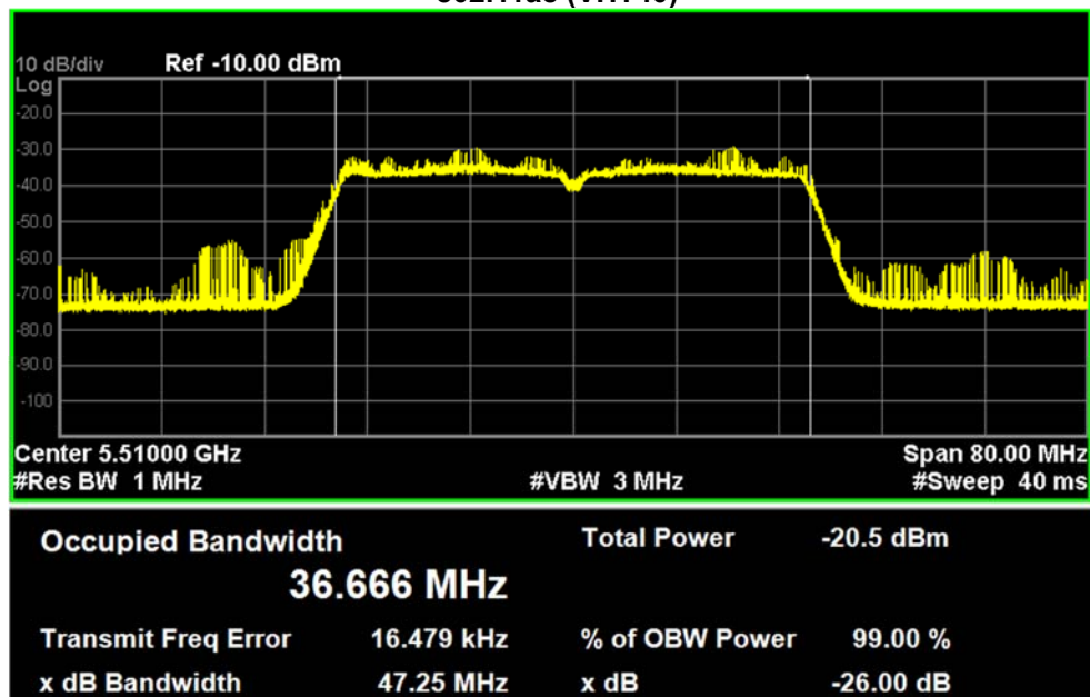
802.11ac (VHT40)
