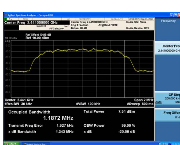
Modulation: \pi/4 DQPSK 2441MHz
