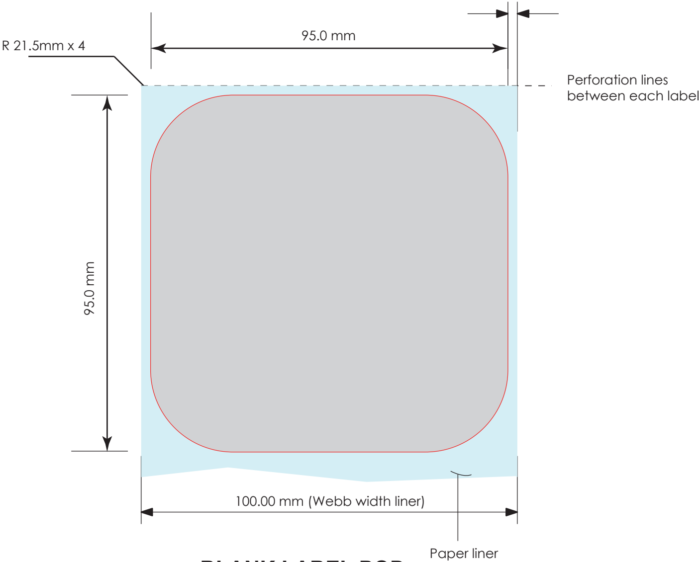
BLANK LABEL POD
