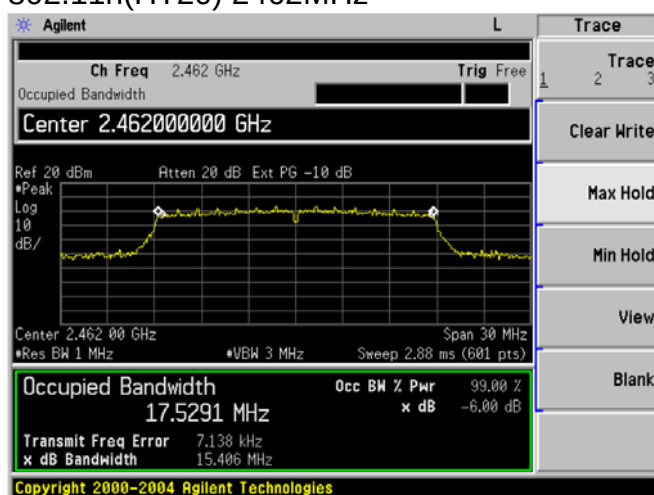
802.11n(HT20) 2462MHz
