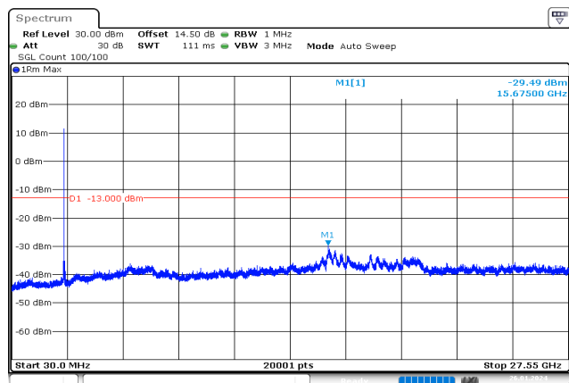
10MHz_Middle_QPSK_50@0 -29.49 dBm
