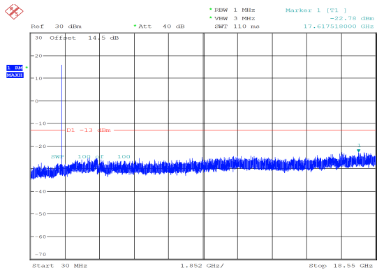
5MHz_Low_QPSK_25@0 -22.78 dBm
