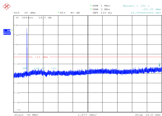
3MHz_Low_QPSK_15@0 -22.35 dBm
