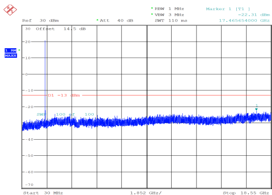
20MHz_Middle_QPSK_1@0 -22.31 dBm
