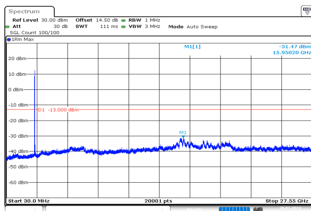
10MHz_Low_QPSK_50@0 -31.47 dBm
