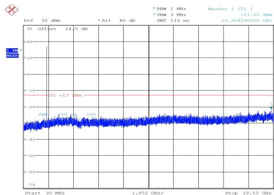
5MHz_Middle_QPSK_25@0 -21.55 dBm
