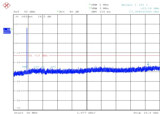
10MHz_Middle_QPSK_50@0 -23.14 dBm
