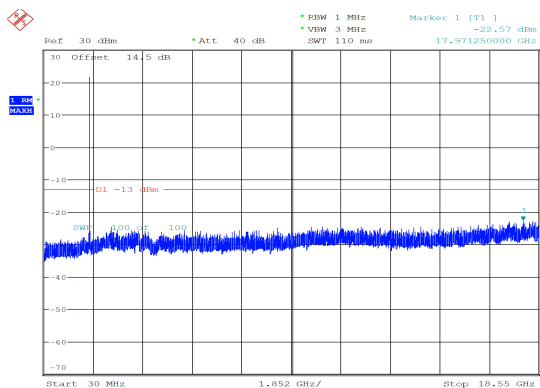
20MHz_Middle_QPSK_1@99 -22.57 dBm
