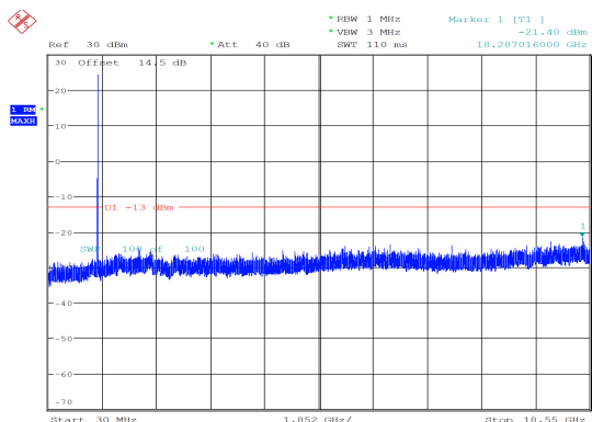
20MHz_Low_QPSK_1@99 -21.40 dBm
