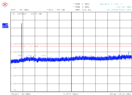
5MHz_Low_QPSK_25@0 -22.40 dBm
