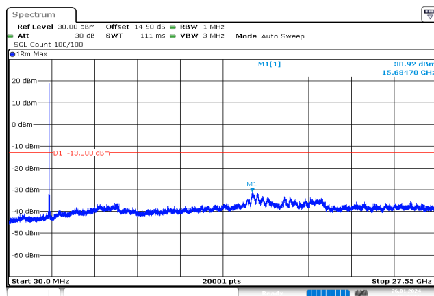
20MHz_Middle_QPSK_1@99 -30.92 dBm
