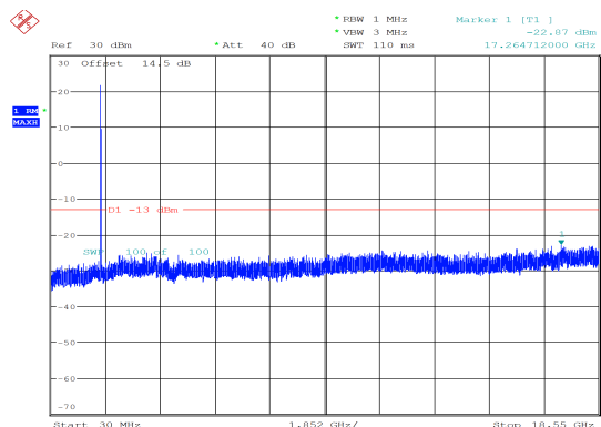
10MHz_Low_QPSK_1@49 -22.87 dBm
