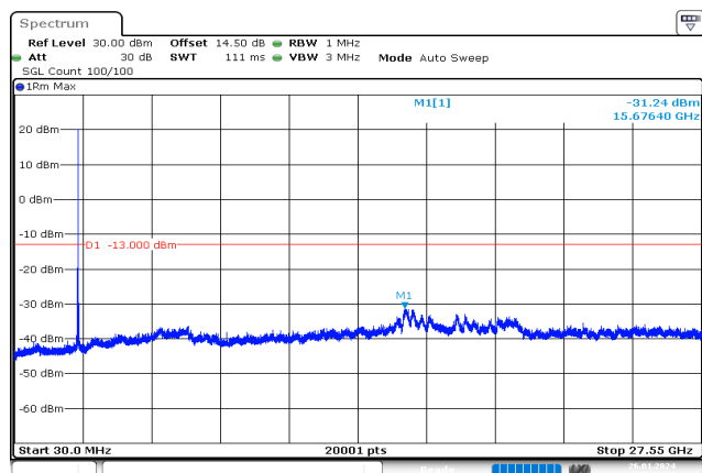
20MHz_Low_QPSK_1@99 -31.24 dBm
