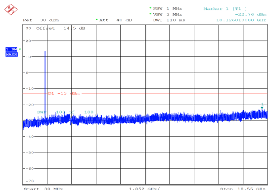
20MHz_Low_QPSK_100@0 -22.76 dBm
