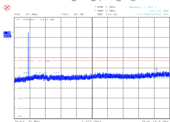
10MHz_Low_QPSK_50@0 -22.26 dBm
