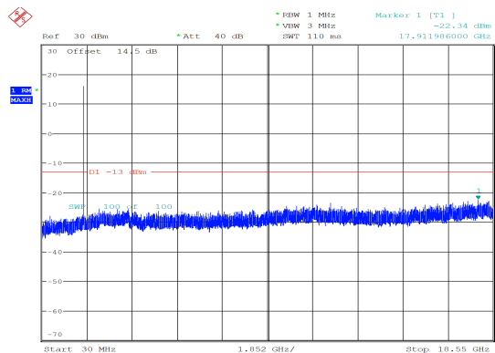
10MHz_Middle_QPSK_50@0 -22.34 dBm
