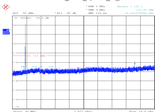
10MHz_Low_QPSK_1@49 -22.38 dBm
