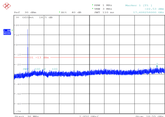
10MHz_Low_QPSK_50@0 -22.53 dBm
