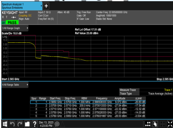
B7 10M 16QAM 50@0 CH 21400
