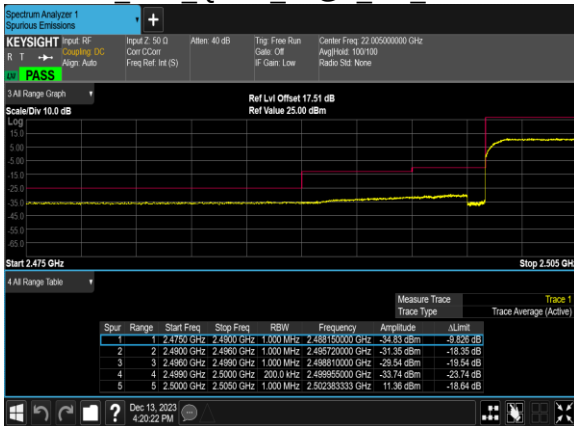
B7 10M 16QAM 50@0 CH 20800
