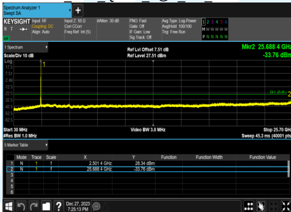
B7 15M QPSK 1@0 CH 21100
