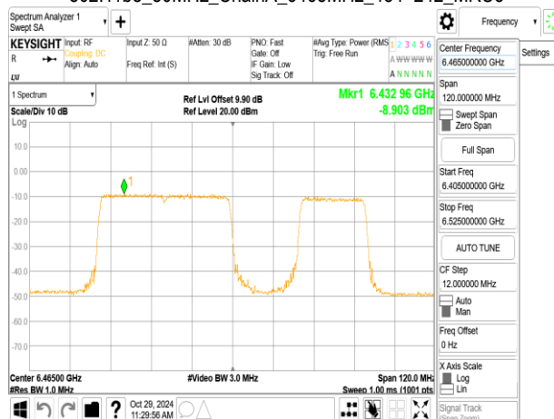
802.11be_80MHz_ChainA_6465MHz_484+242_MRU4
