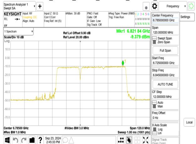
802.11be_80MHz_ChainA_6785MHz_484+242_MRU3
