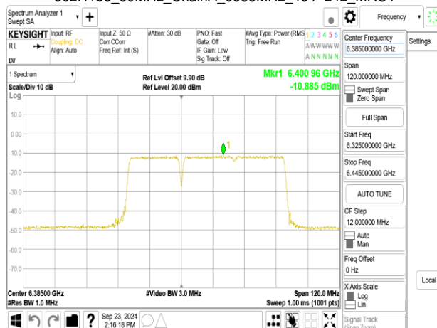
802.11be_80MHz_ChainA_6385MHz_484+242_MRU3
