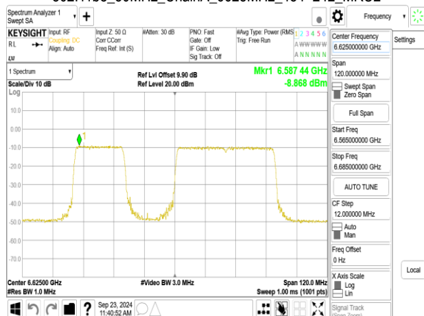
802.11be_80MHz_ChainA_6625MHz_484+242_MRU4
