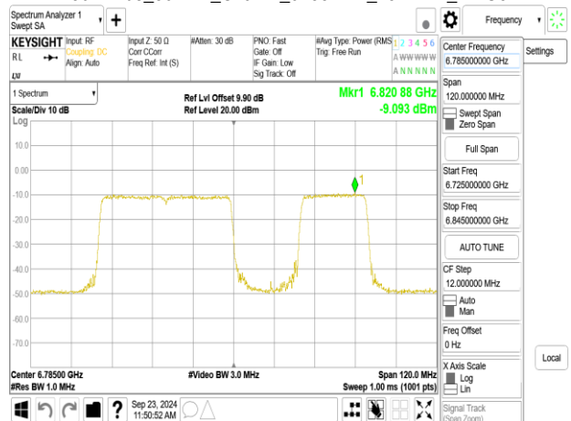
802.11be_80MHz_ChainA_6785MHz_RU484_66
