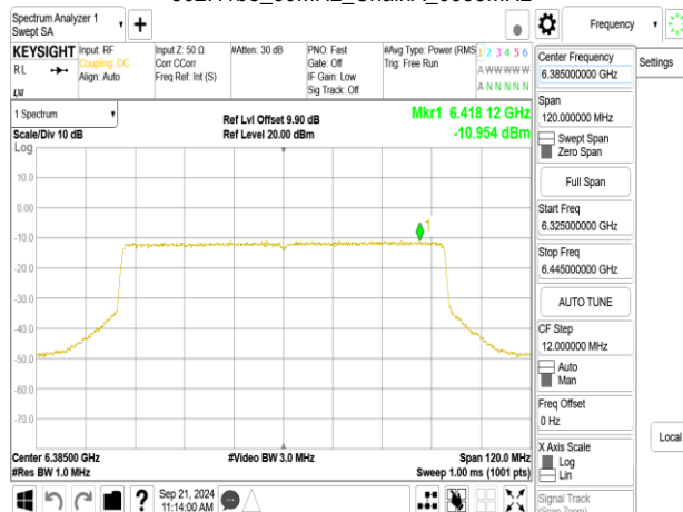
802.11be_80MHz_ChainA_6385MHz_484+242_MRU1
