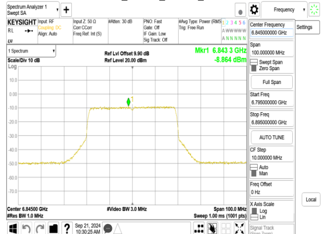
802.11be_40MHz_ChainA_6845MHz
