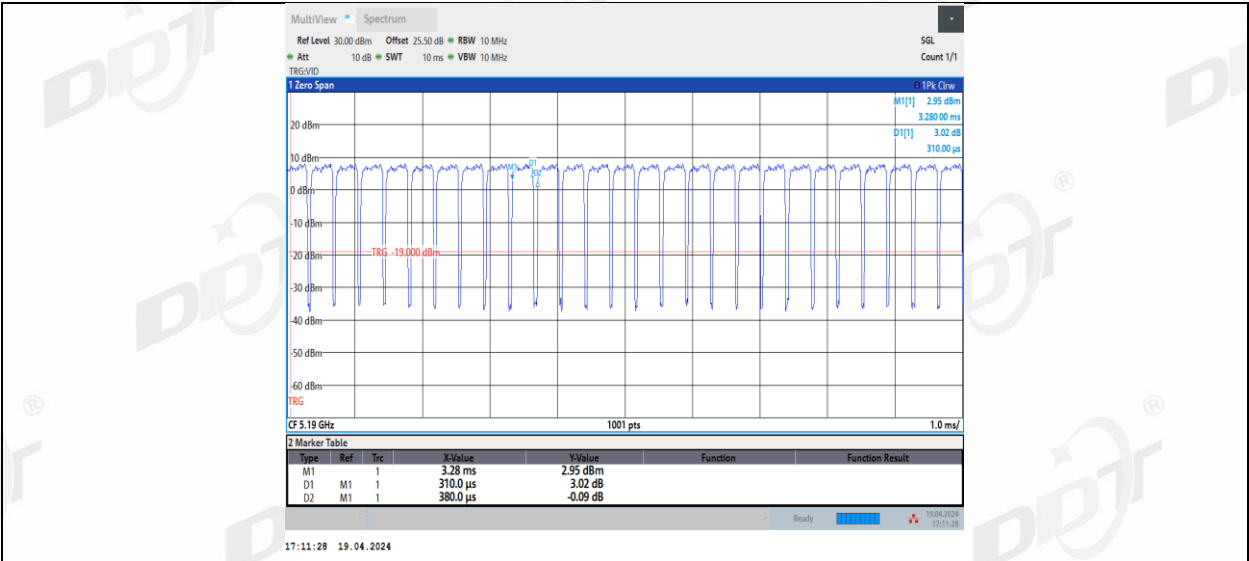
11BE40MIMO_Ant2_5190
