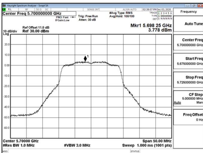
802.11n_20MHz_CH1_5700MHz-5700
