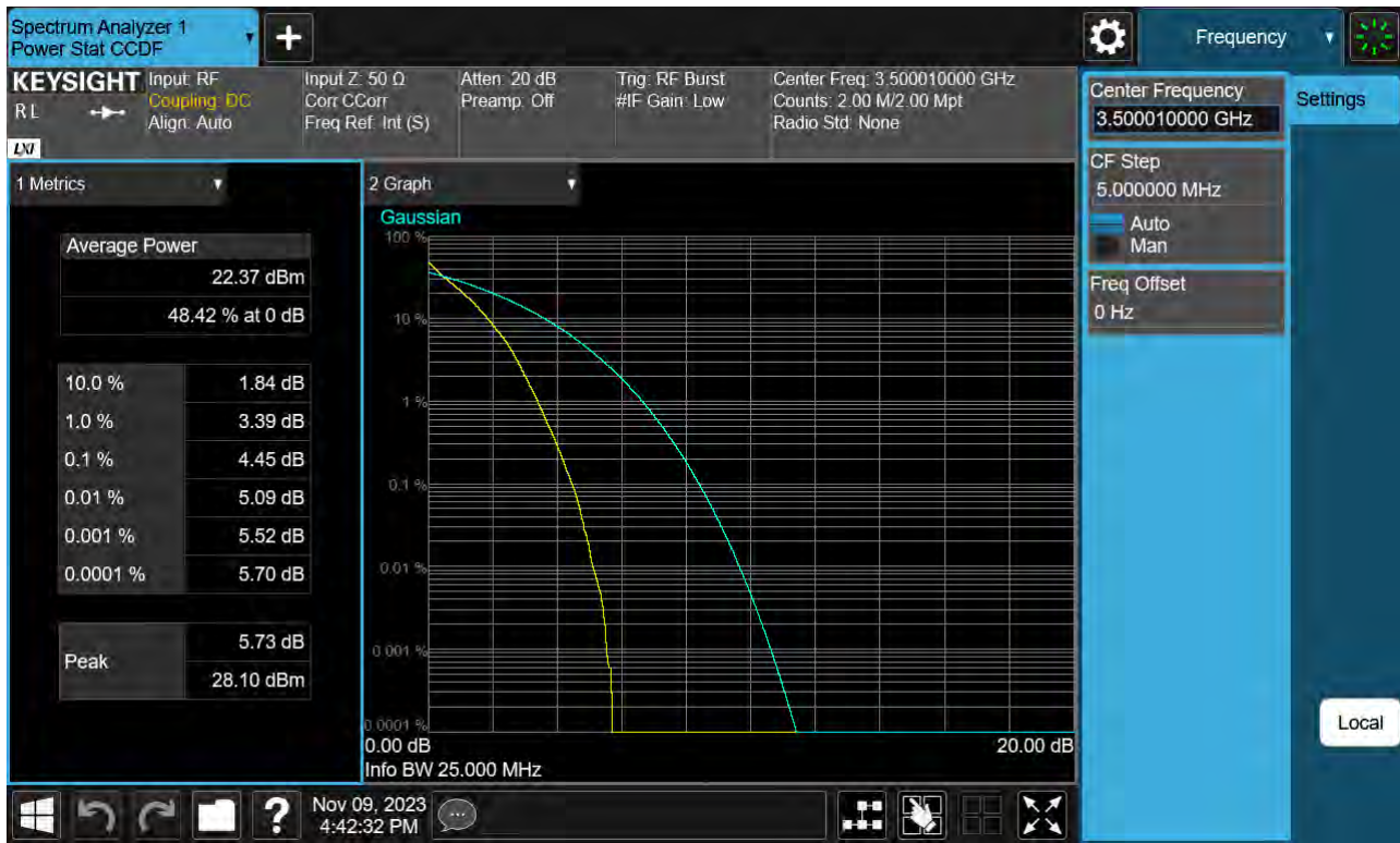
Sub6 n77(78). PAR Plot (25 M BW_Ch.633334_ BPSK)
