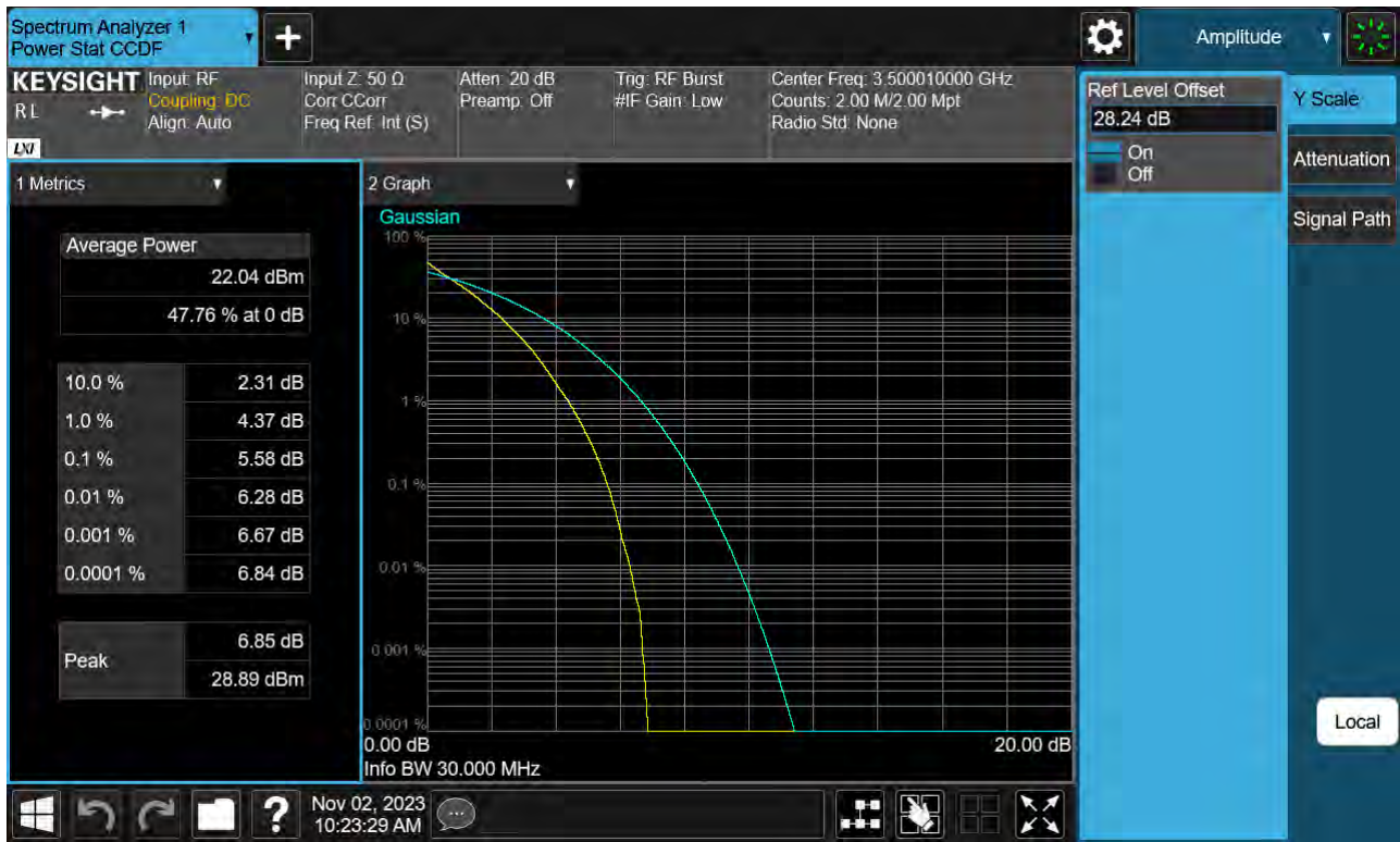
Sub6 n77(78). PAR Plot (30 M BW_Ch.633334_QPSK)
