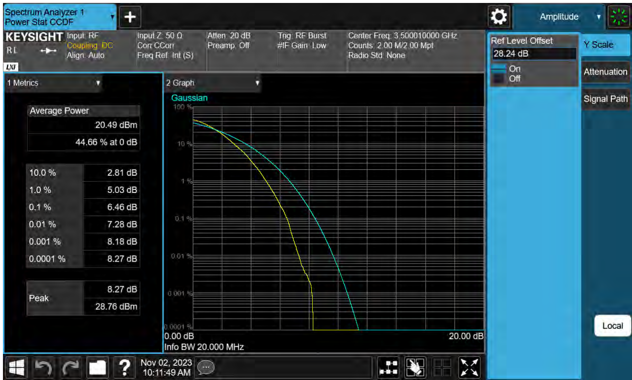
Sub6 n77(78). PAR Plot (20 M BW_Ch.633334_64QAM)
