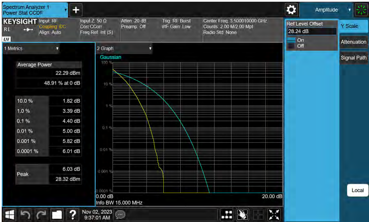
Sub6 n77(78). PAR Plot (15 M BW_Ch.633334_ BPSK)
