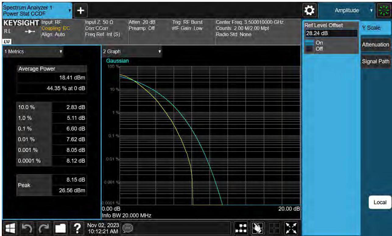
Sub6 n77(78). PAR Plot (20 M BW_Ch.633334_256QAM)
