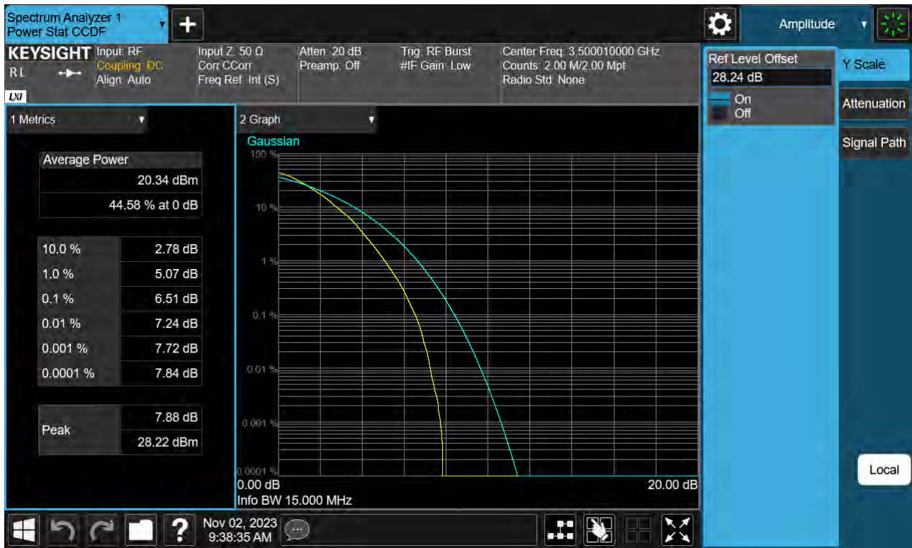
Sub6 n77(78). PAR Plot (15 M BW_Ch.633334_64QAM)
