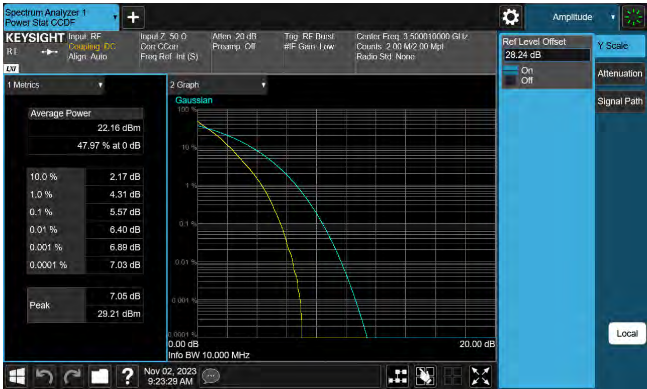
Sub6 n77(78). PAR Plot (10 M BW_Ch.633334_QPSK)
