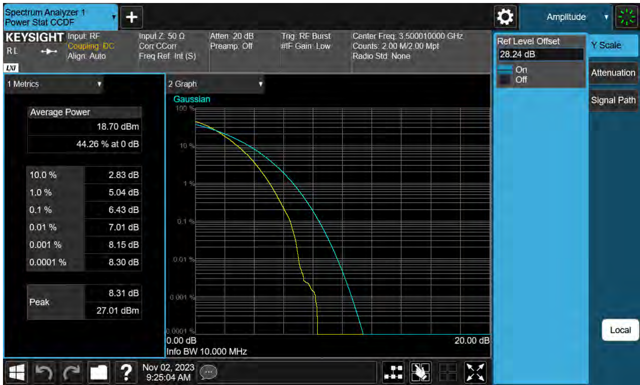
Sub6 n77(78). PAR Plot (10 M BW_Ch.633334_256QAM)
