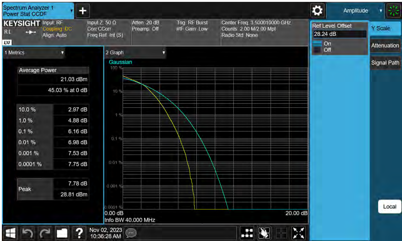
Sub6 n77(78). PAR Plot (40 M BW_Ch.633334_16QAM)
