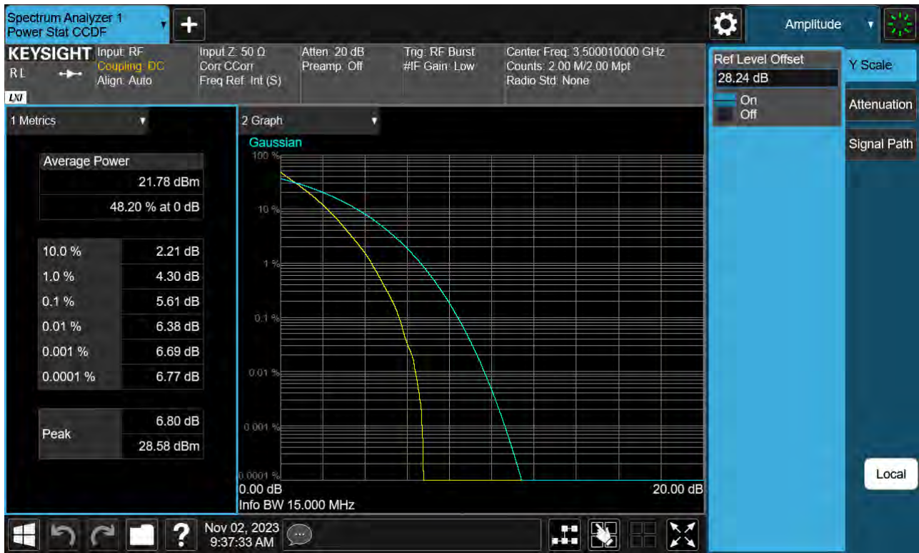
Sub6 n77(78). PAR Plot (15 M BW_Ch.633334_QPSK)
