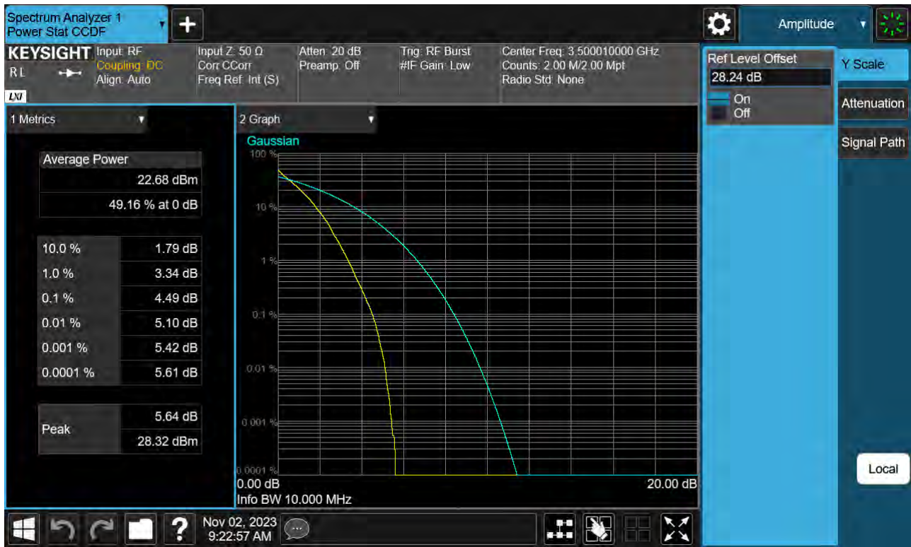
Sub6 n77(78). PAR Plot (10 M BW_Ch.633334_ BPSK)
