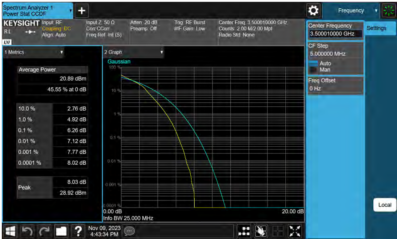
Sub6 n77(78). PAR Plot (25 M BW_Ch.633334_16QAM)
