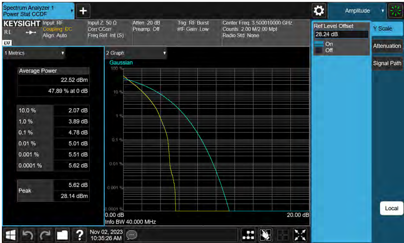
Sub6 n77(78). PAR Plot (40 M BW_Ch.633334_ BPSK)
