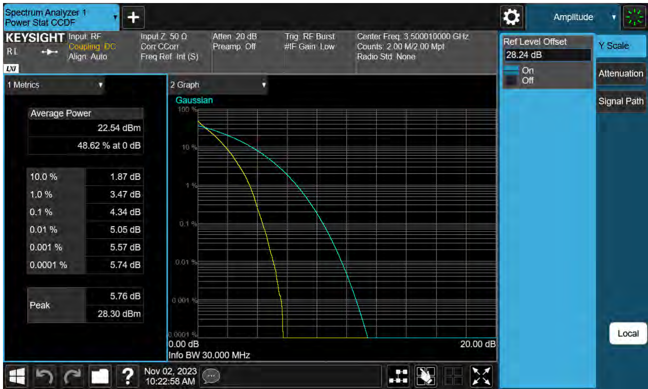
Sub6 n77(78). PAR Plot (30 M BW_Ch.633334_ BPSK)
