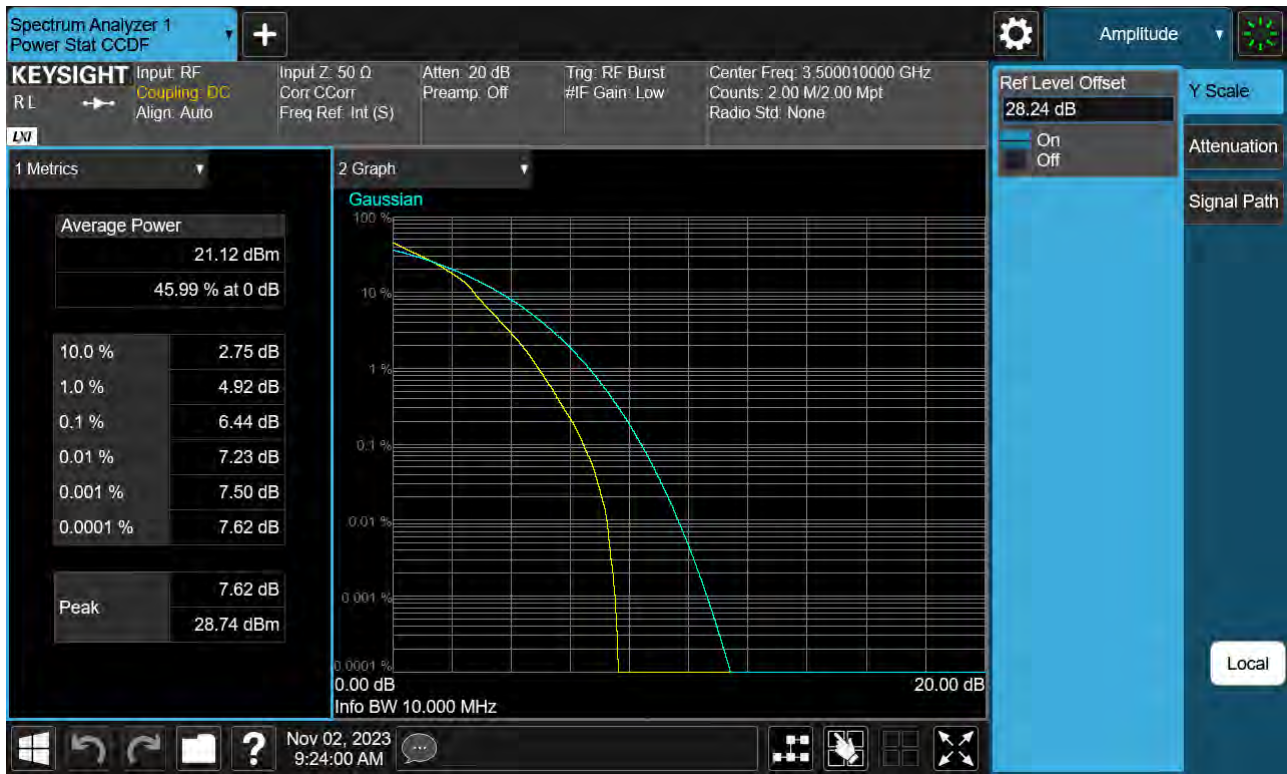
Sub6 n77(78). PAR Plot (10 M BW_Ch.633334_16QAM)
