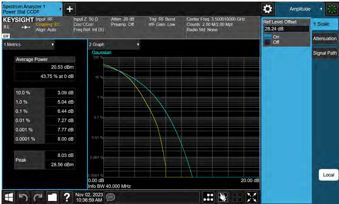
Sub6 n77(78). PAR Plot (40 M BW_Ch.633334_64QAM)
