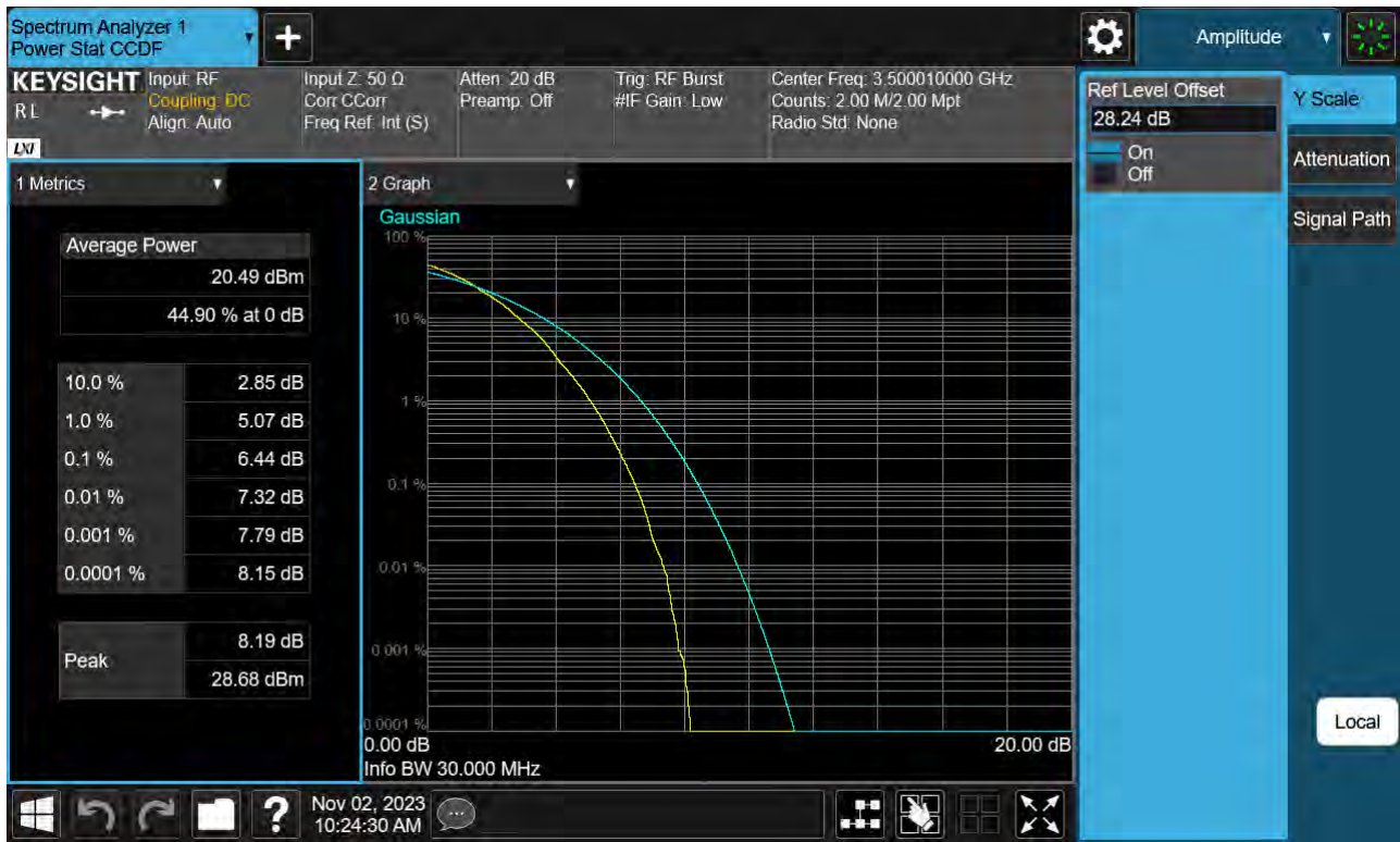
Sub6 n77(78). PAR Plot (30 M BW_Ch.633334_64QAM)
