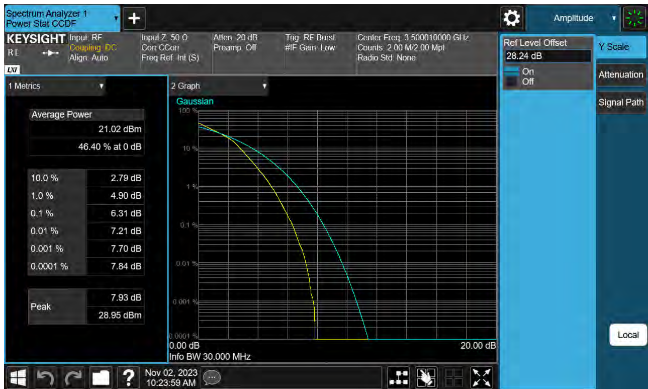
Sub6 n77(78). PAR Plot (30 M BW_Ch.633334_16QAM)
