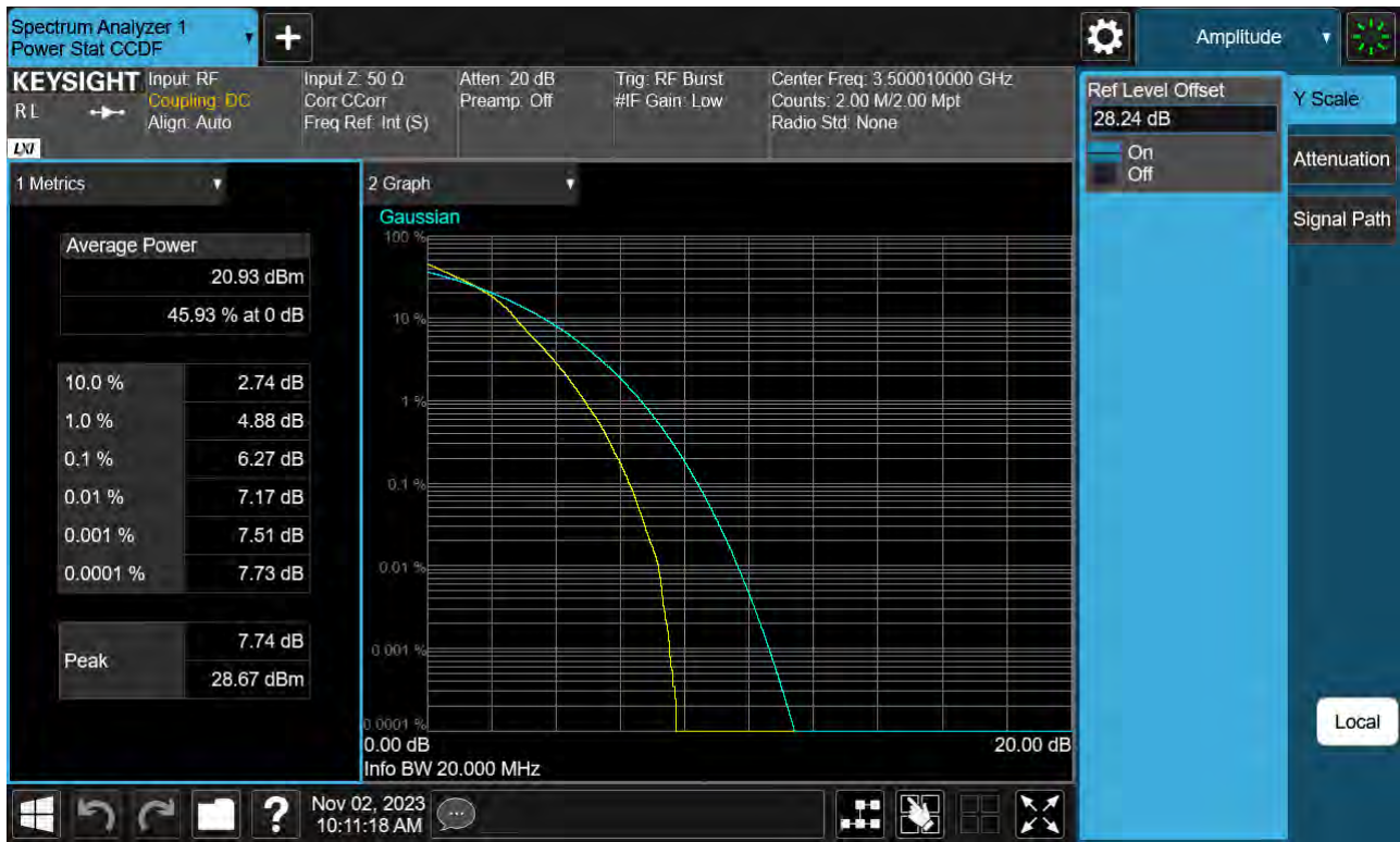
Sub6 n77(78). PAR Plot (20 M BW_Ch.633334_16QAM)
