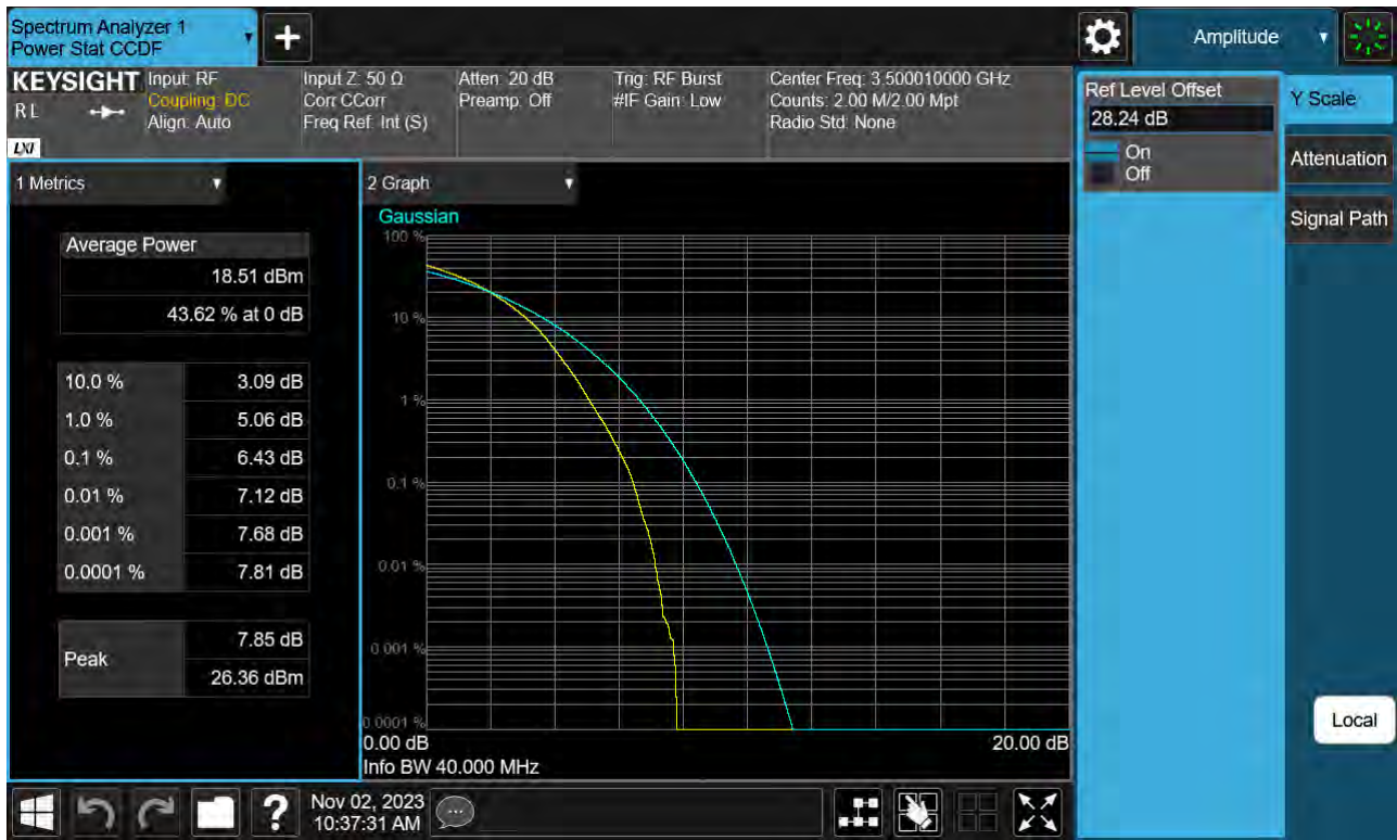
Sub6 n77(78). PAR Plot (40 M BW_Ch.633334_256QAM)
