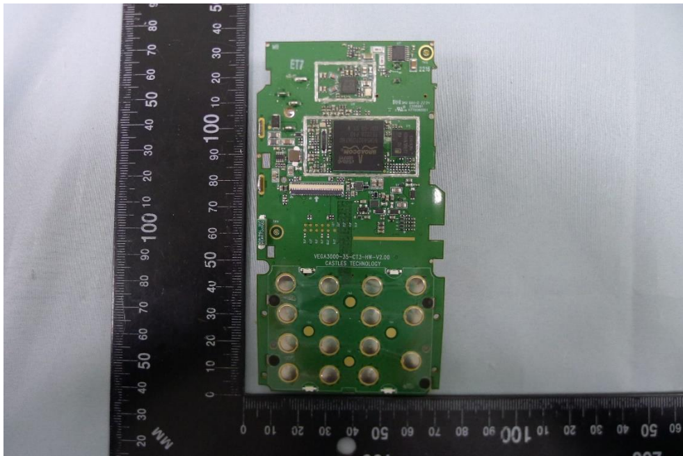
(24) EUT Photos
