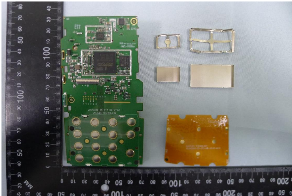
(23) EUT Photos
