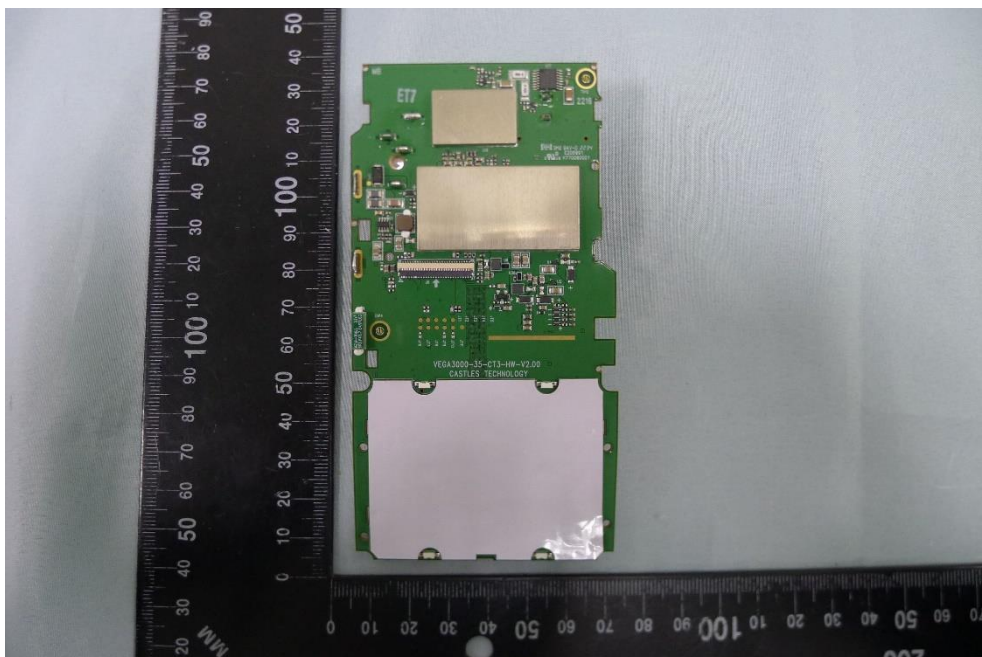
(22) EUT Photos
