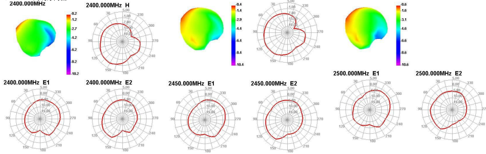
2.4G WIFI天线方向图
