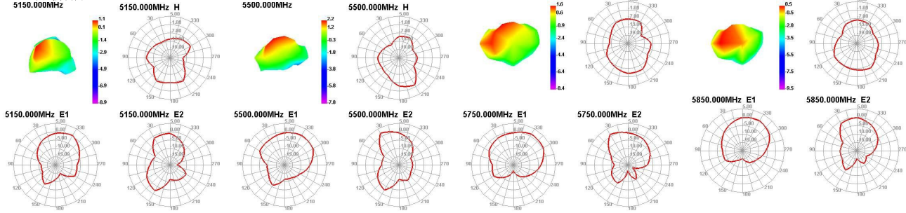
5G WIFI天线方向图
