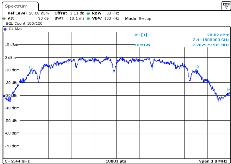
OBW 2440MHz Ant1
