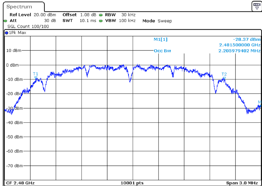
OBW 2480MHz Ant1
