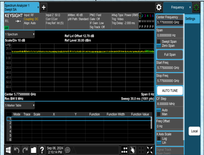
NTNV-11AC80SISO-Ant4-5775
