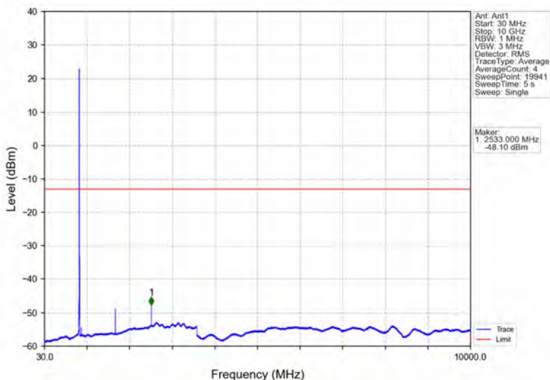
Band5_5MHz_QPSK_HCH_846.5MHz_RB_1_24_NTNV
