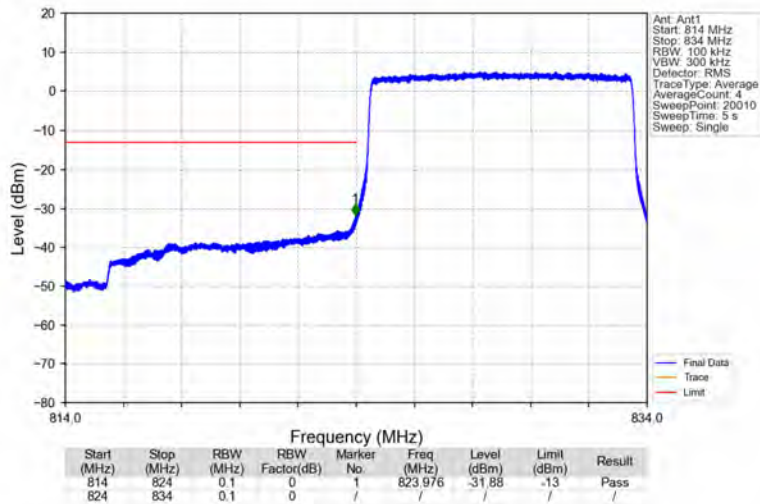
Band5_10MHz_QPSK_LCH_829MHz_RB_50_0_NTNV
