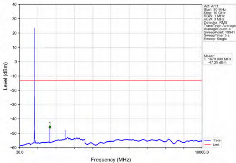
Band5_10MHz_QPSK_HCH_844MHz_RB_1_49_NTNV
