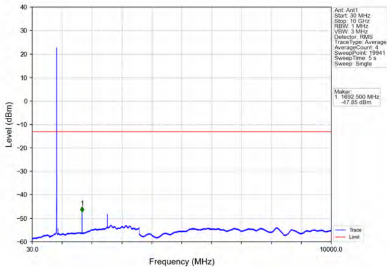
Band5_3MHz_QPSK_HCH_847.5MHz_RB_1_14_NTNV
