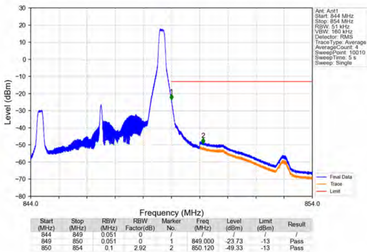
Band5_5MHz_QPSK_HCH_846.5MHz_RB_1_24_NTNV
