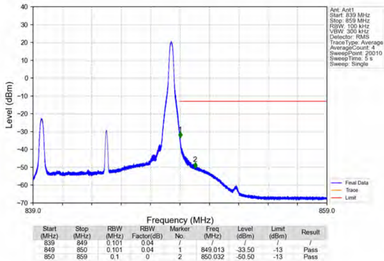
Band5_10MHz_QPSK_HCH_844MHz_RB_1_49_NTNV
