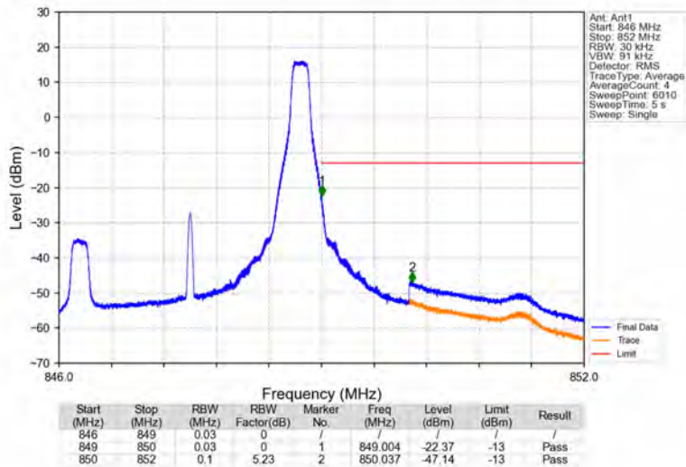
Band5_3MHz_QPSK_HCH_847.5MHz_RB_1_14_NTNV
