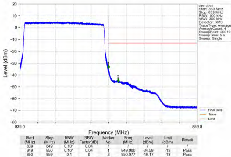
Band5_10MHz_QPSK_HCH_844MHz_RB_50_0_NTNV
