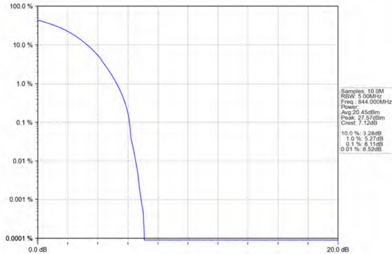
Band5_10MHz_QPSK_HCH_844MHz_RB_50_0_NTNV
