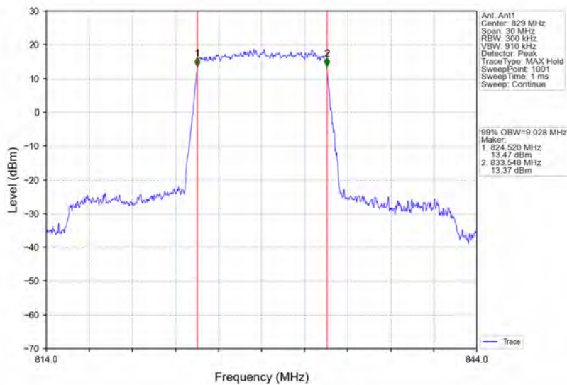
Band5_10MHz_QPSK_LCH_829MHz_RB_50_0_NTNV
