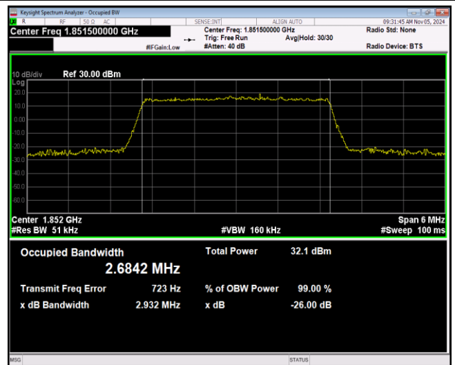
Band2-3MHz-QPSK-19185-15RB#0
