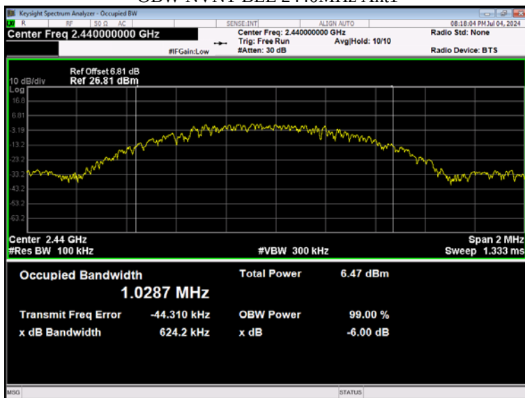
OBW NVNT BLE 2440MHz Ant1
