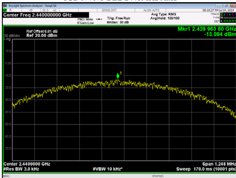
PSD NVNT BLE 2440MHz Ant1
