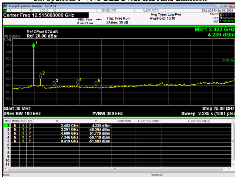
Tx. Spurious NVNT BLE 2402MHz Ant1 Emission
