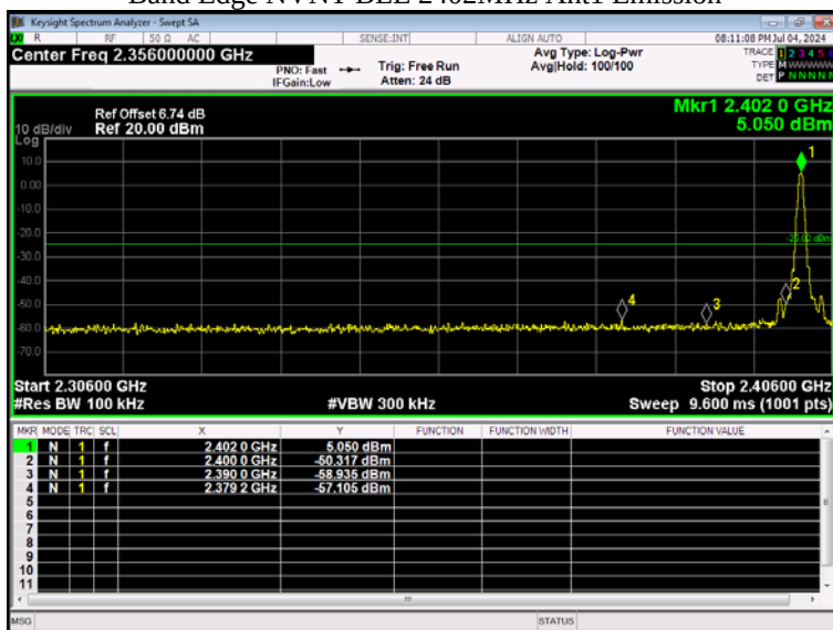
Band Edge NVNT BLE 2402MHz Ant1 Emission
