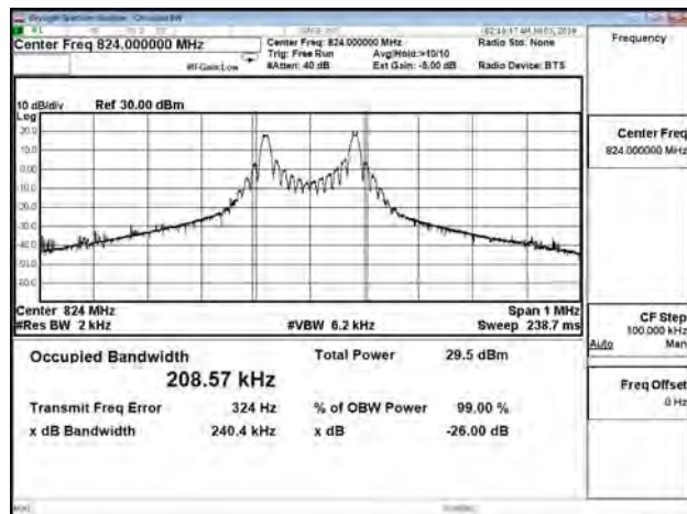
B26_15K_CH26790_BPSK_1RB11
