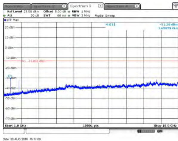
B26_15K_CH26788_QPSK_3RB3_above 1G
