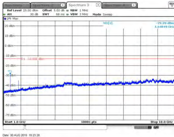
B26_15K_CH26915_QPSK_3RB3_above 1G
