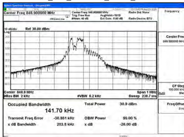
B26_15K_CH27039_QPSK_3RB3
