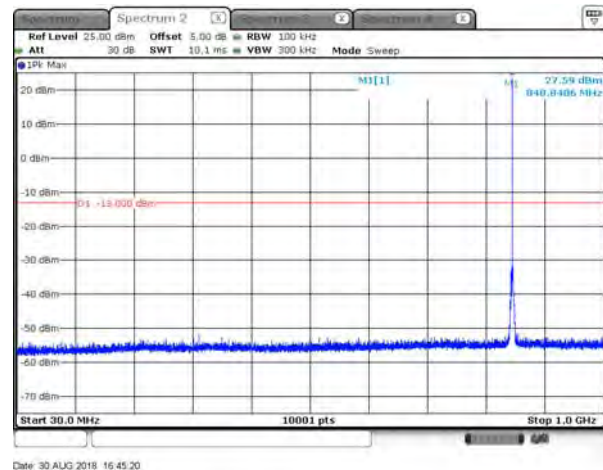
B26_15K_CH27039_QPSK_3RB3_under 1G
