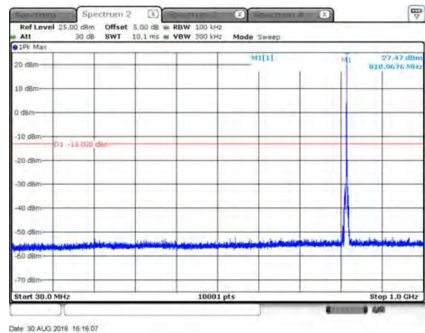
B26_15K_CH26788_QPSK_3RB3_under 1G
