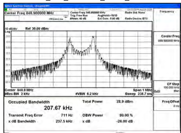
B26_15K_CH27039_BPSK_1RB11
