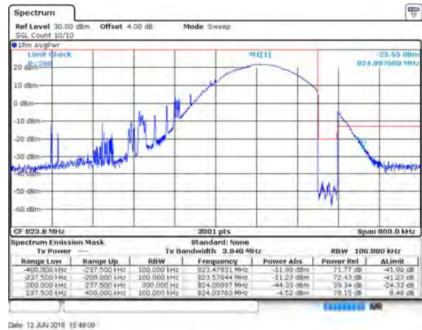
B26_15K_CH26788_QPSK_1RB11
