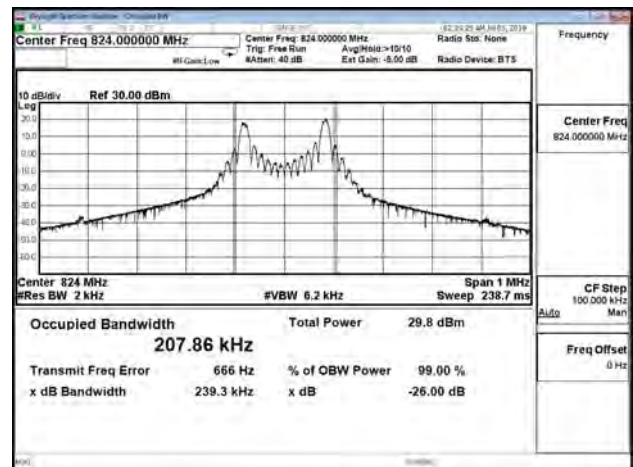
B26_15K_CH26790_QPSK_1RB11
