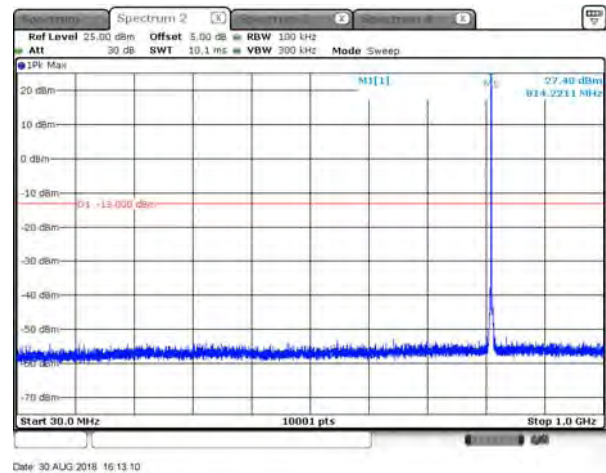
B26_15K_CH26740_QPSK_3RB3_under 1G
