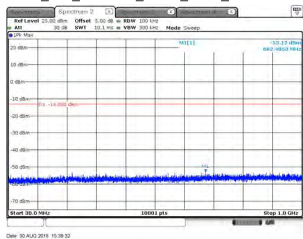
B4_15K_CH20399_QPSK_3RB3_under 1G
