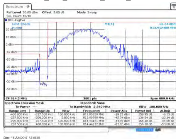
B26_15K_CH26692_QPSK_3RB3
