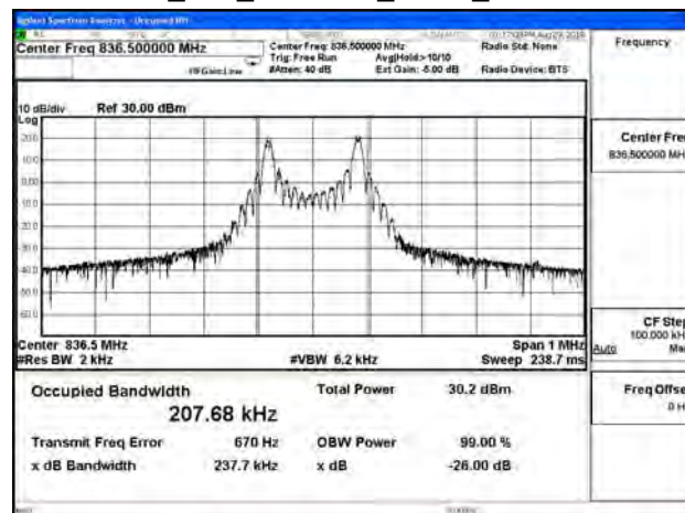
B5_15K_CH20525_BPSK_1RB11
