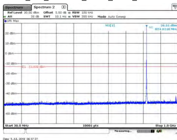
B26_15K_CH26790_QPSK_3RB3_under 1G
