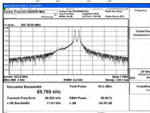
B26_3.75K_CH26788_BPSK_1RB47
