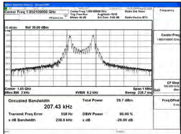
B2_15K_CH18601_BPSK_1RB11
