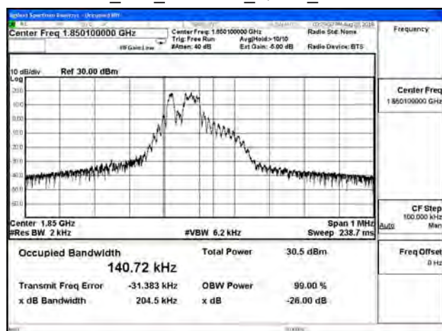
B2_15K_CH18601_QPSK_3RB3
