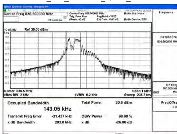
B26_15K_CH26915_QPSK_3RB3
