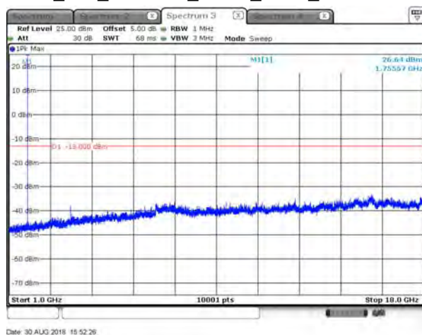
B4_15K_CH20399_QPSK_3RB3_above 1G
