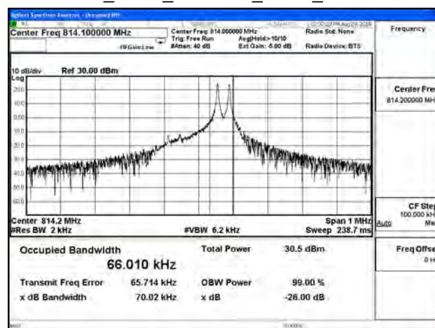
B26_3.75K_CH26692_BPSK_1RB47
