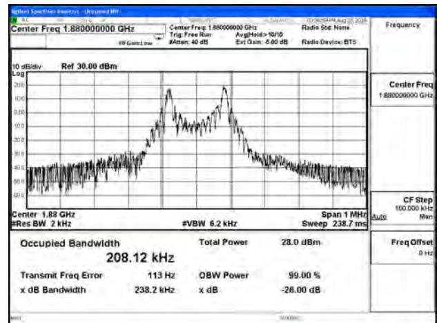
B2_15K_CH18900_BPSK_1RB11
