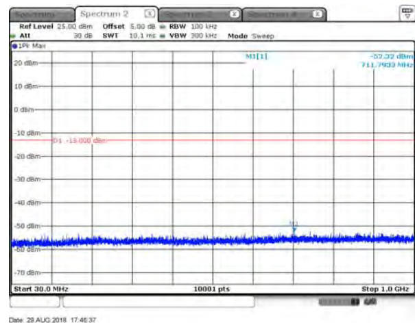
B2_15K_CH19199_QPSK_3RB3_under 1G
