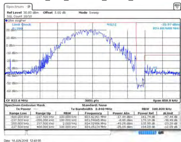
B26_15K_CH26788_QPSK_3RB3
