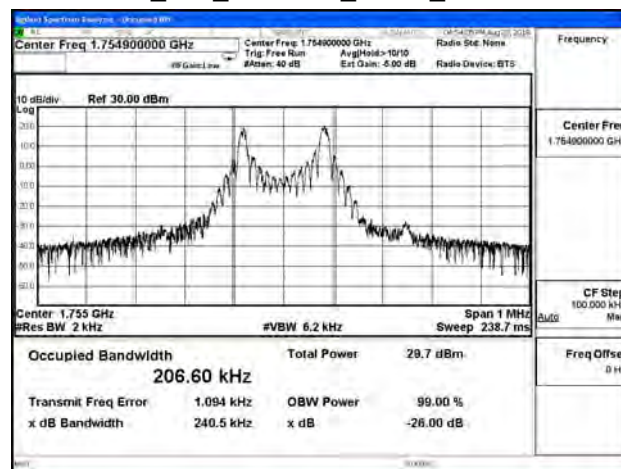
B4_15K_CH20399_QPSK_1RB11
