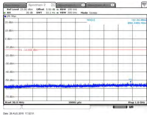
B2_15K_CH19199_QPSK_3RB3_under 1G
