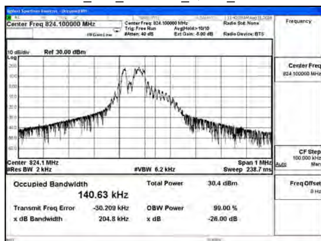
B26_15K_CH26791_QPSK_3RB3
