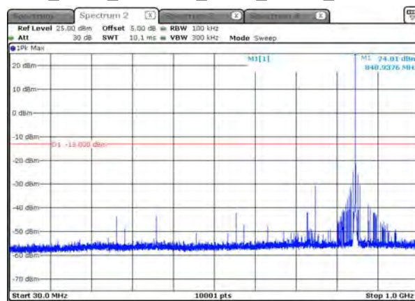
B26_3.75K_CH27039_BPSK_1RB47_under 1G
