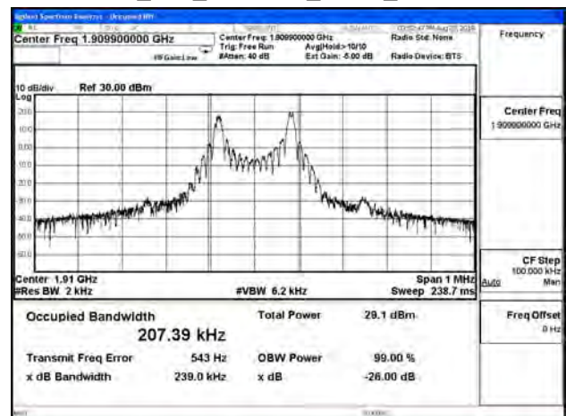
B2_15K_CH19199_BPSK_1RB11
