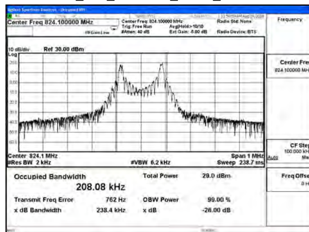
B5_15K_CH20401_BPSK_1RB11
