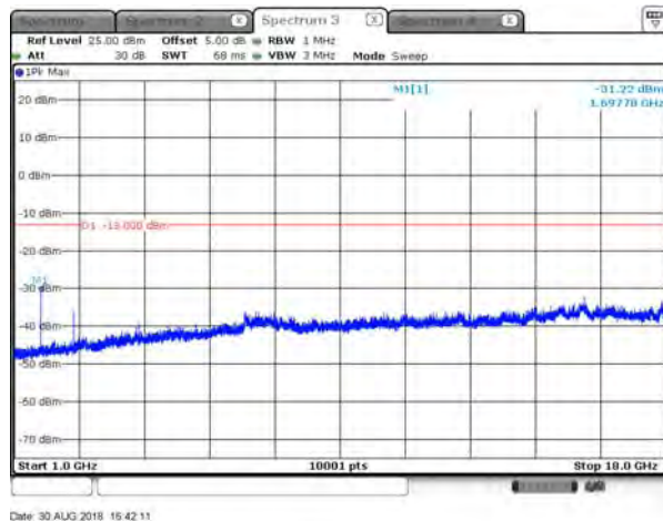
B26_15K_CH27039_QPSK_3RB3_above 1G
