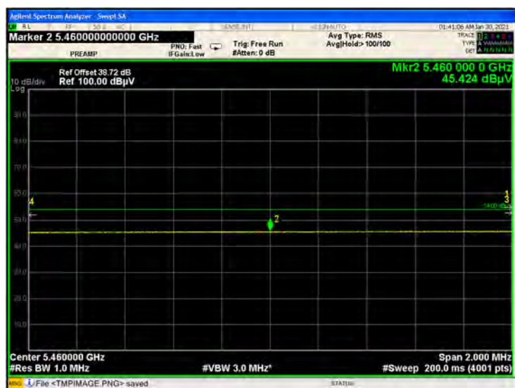
U-NII-2C 11n20 CH100 AV
