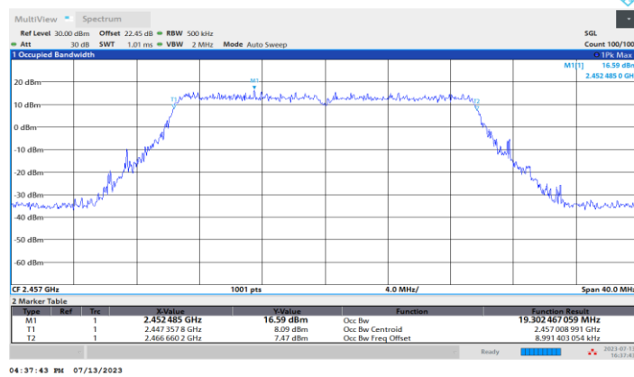
11BE20MIMO_Ant4_2457
