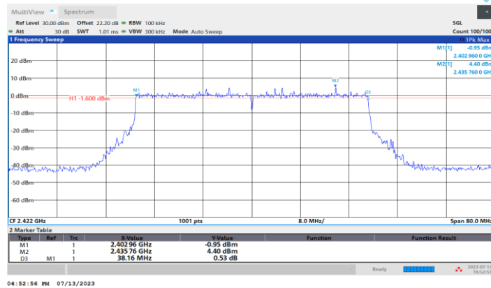
11BE40MIMO_Ant3_2422
