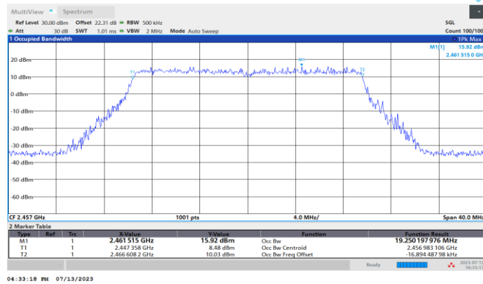
11BE20MIMO_Ant1_2457
