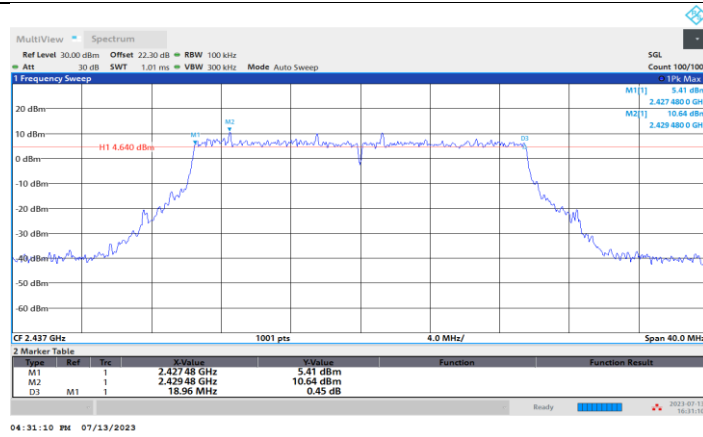
11BE20MIMO_Ant4_2437
