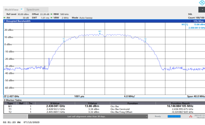
11B-CDD_Ant3_2437
