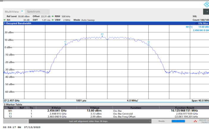
11B-CDD_Ant1_2457
