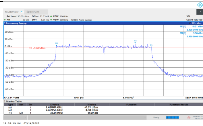
11BE40MIMO_Ant1_2447
