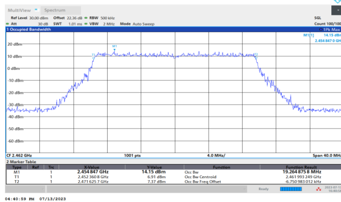
11BE20MIMO_Ant1_2462
