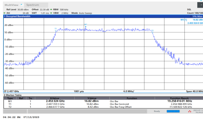
11BE20MIMO_Ant2_2457
