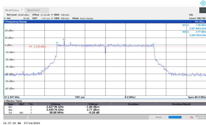
11BE40MIMO_Ant3_2447
