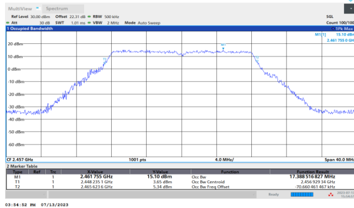
11G-CDD_Ant1_2457
