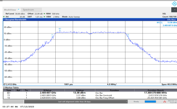
11G-CDD_Ant2_2412
