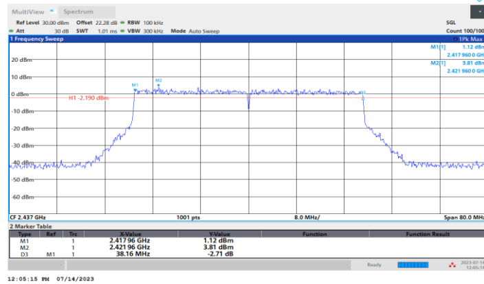
11BE40MIMO_Ant3_2437
