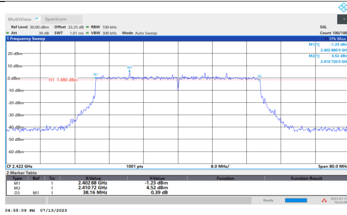
11BE40MIMO_Ant4_2422
