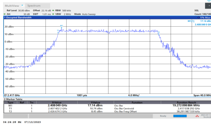
11BE20MIMO_Ant4_2417
