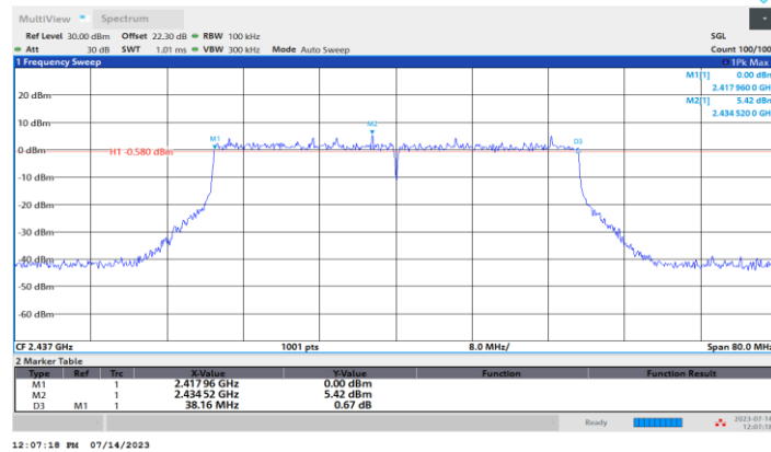
11BE40MIMO_Ant4_2437
