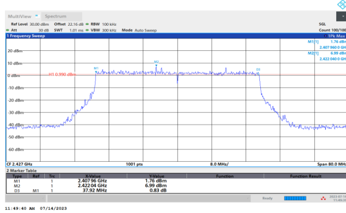
11BE40MIMO_Ant1_2427
