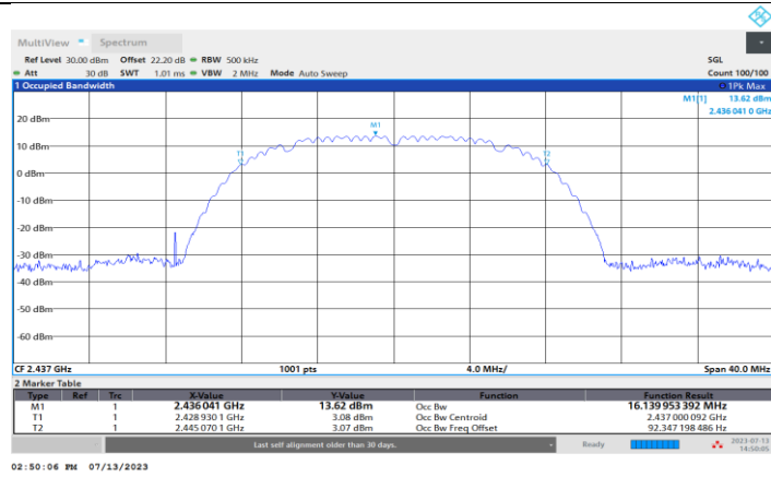
11B-CDD_Ant2_2437
