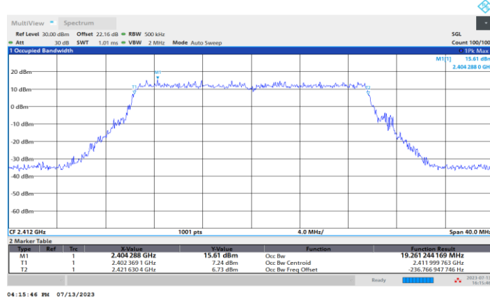
11BE20MIMO_Ant4_2412
