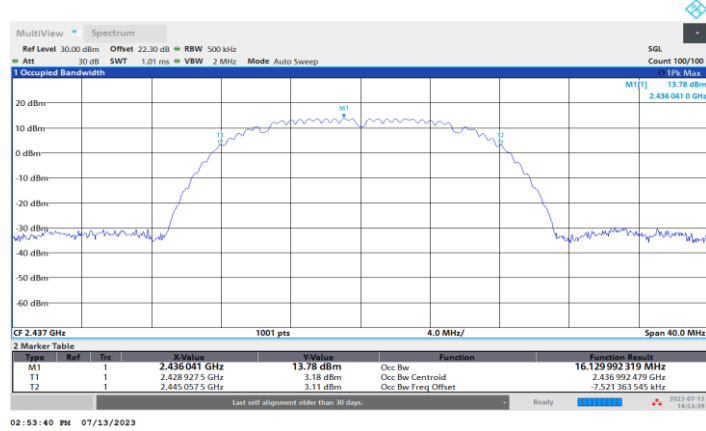
11B-CDD_Ant4_2437
