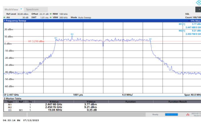
11BE20MIMO_Ant1_2457
