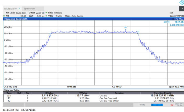
11BE20MIMO_Ant1_2412
