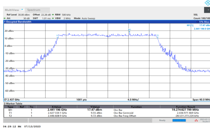
11BE20MIMO_Ant3_2437
