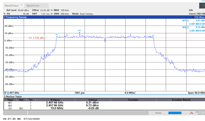
11BE20MIMO_Ant4_2457
