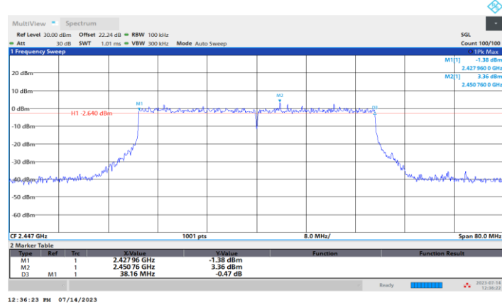
11BE40MIMO_Ant2_2447
