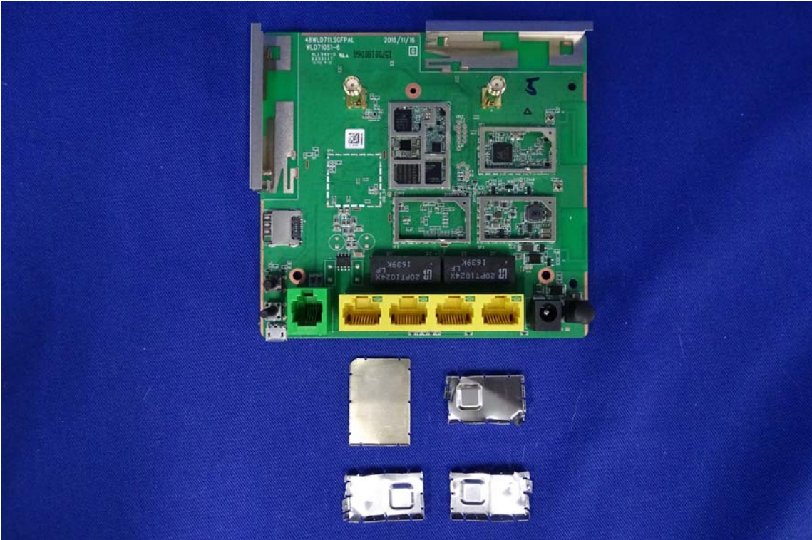
(8) EUT Photo (Antenna)
