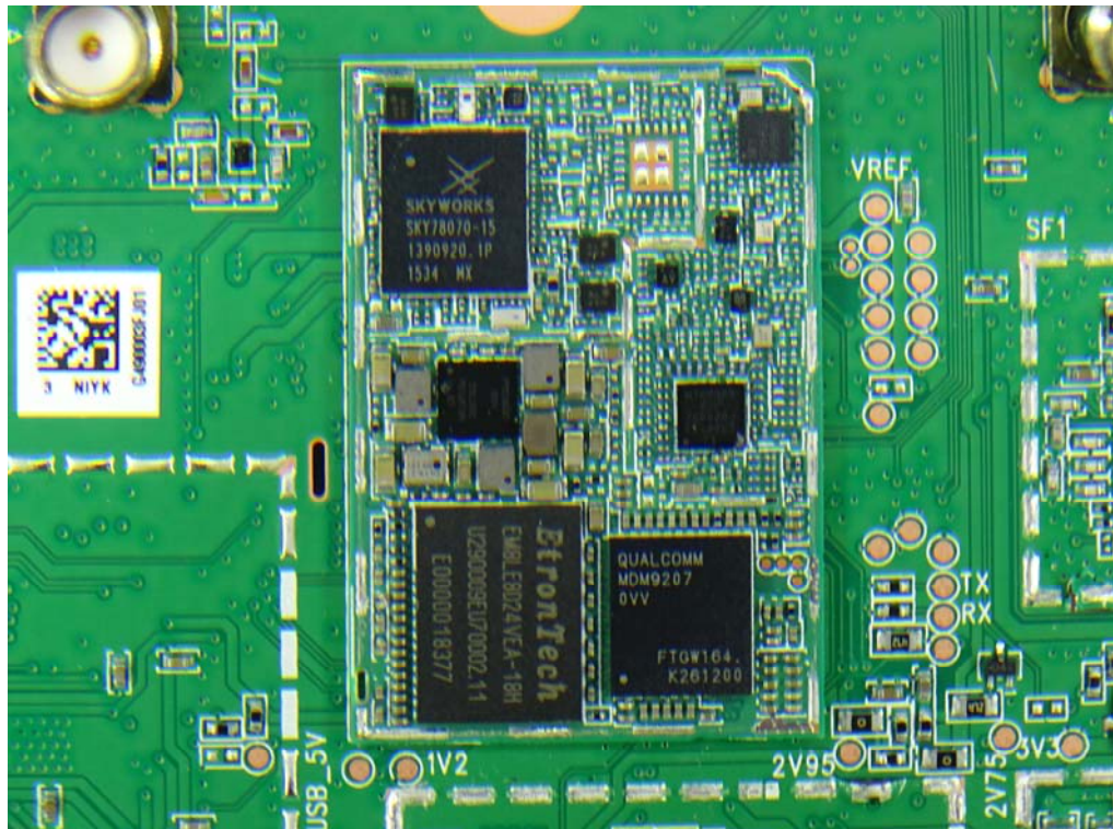
(10) EUT Photo
