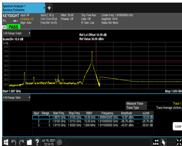
Band2-20MHz-16QAM-19100-1RB#99
