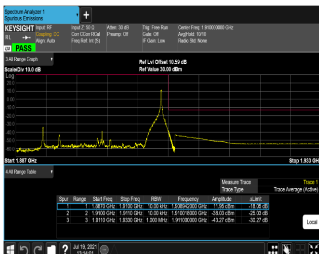
Band2-20MHz-QPSK-19100-1RB#99
