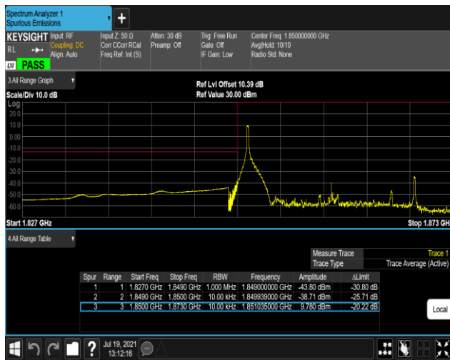
Band2-20MHz-16QAM-18700-100RB#0
