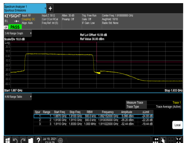
Band2-20MHz-QPSK-19100-100RB#0
