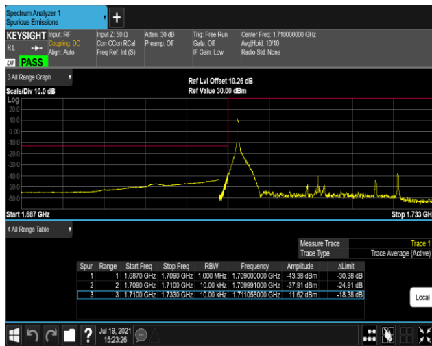
Band4-20MHz-QPSK-20050-100RB#0
