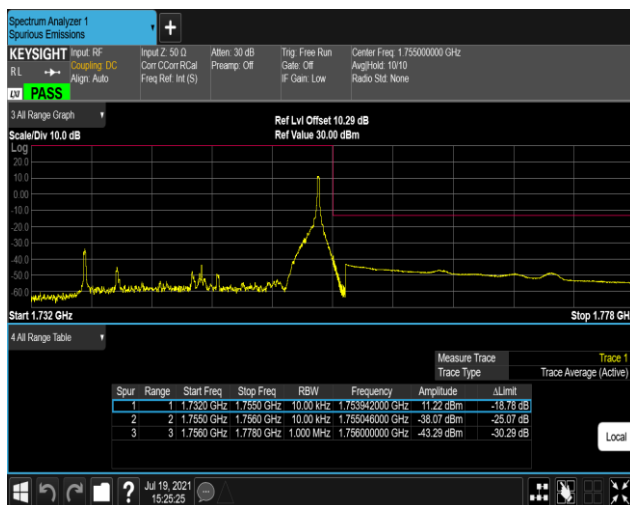
Band4-20MHz-QPSK-20300-1RB#99
