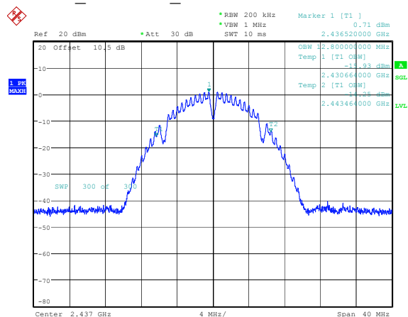
b 2437MHz Chain 1 12.800MHz
