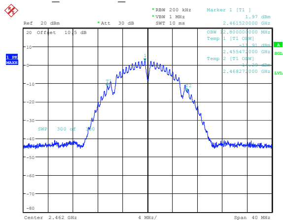
b 2462MHz Chain 0 12.800MHz
