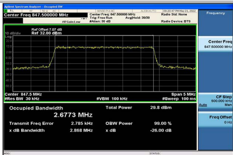
Band5-3MHz-QPSK-20635-15RB#0-2.6773
