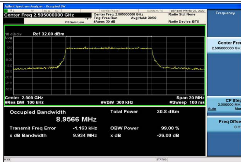
Band7-10MHz-QPSK-20800-50RB#0-8.9566
