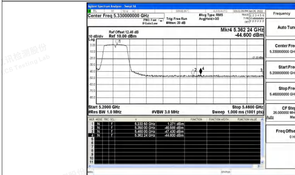
11AC80SISO_Ant0_Low_5210_AV
