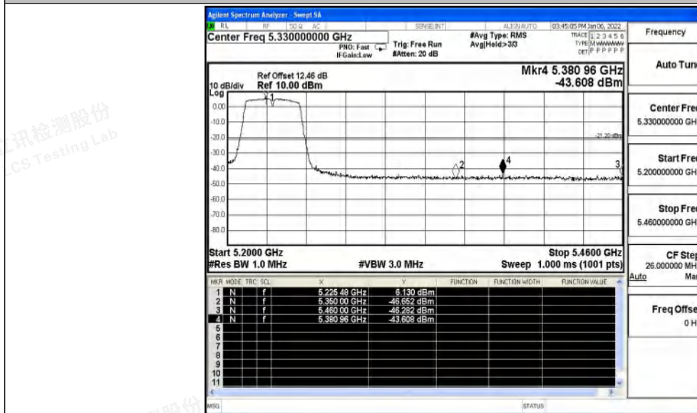
11AC80SISO_Ant1_Low_5210_AV
