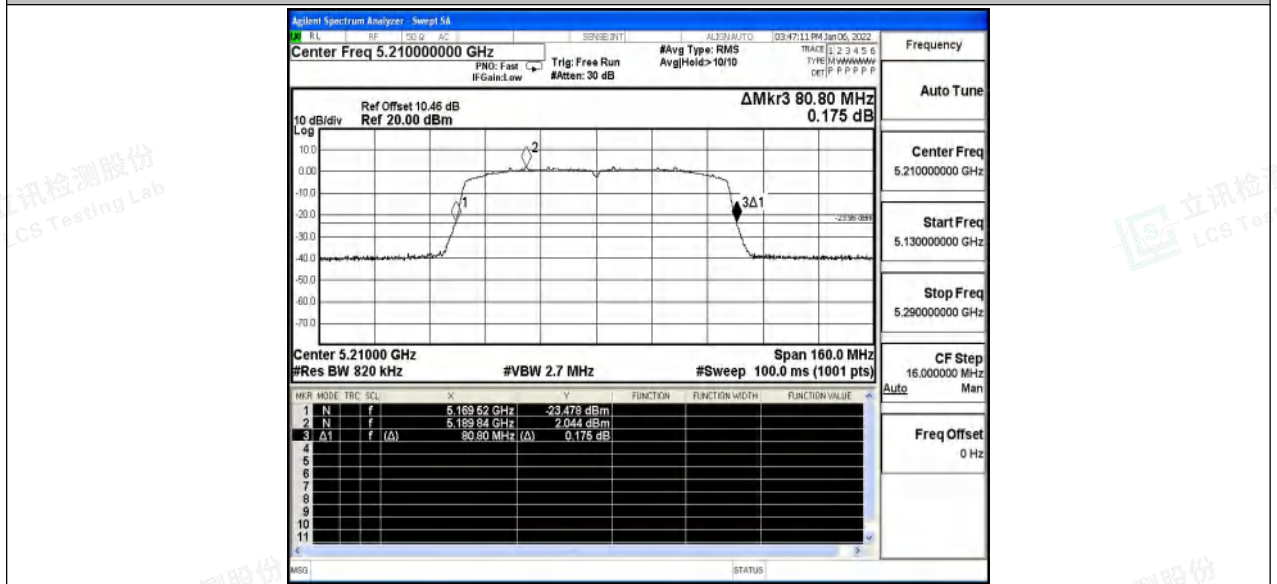
11AC80SISO_Ant1_5210
