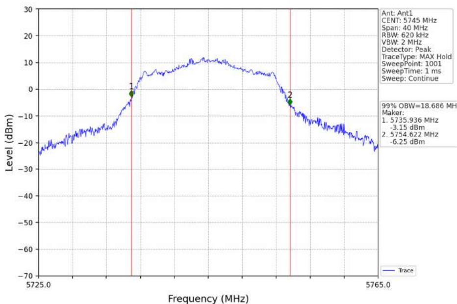
802.11a LCH_5745MHz_Ant1_NTNV
