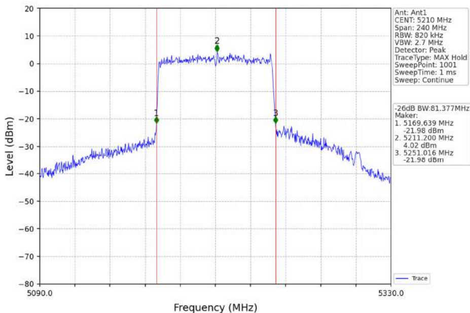
802.11ax(HEW80) MCH_5210MHz_RU996_Left_Ant1_NTNV
