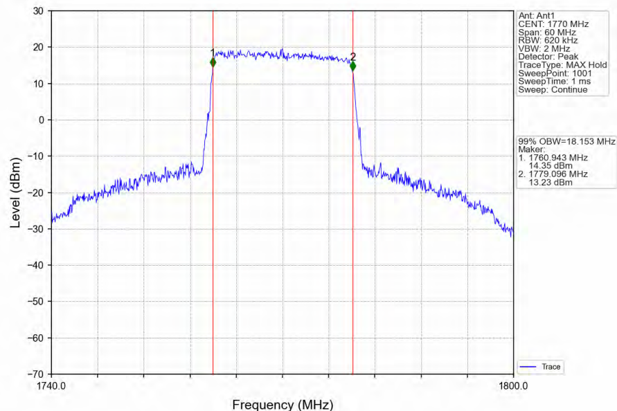
Band66_20MHz_QPSK_HCH_1770MHz_RB_100_0_NTNV
