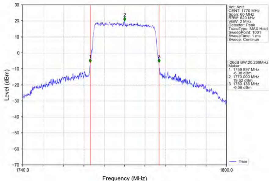
Band66_20MHz_QPSK_HCH_1770MHz_RB_100_0_NTNV
