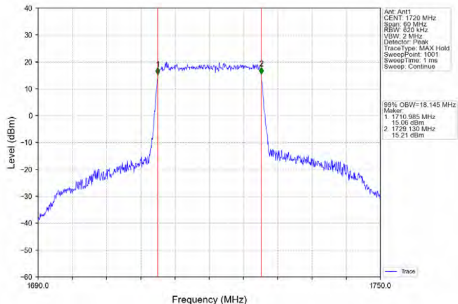
Band66_20MHz_QPSK_LCH_1720MHz_RB_100_0_NTNV
