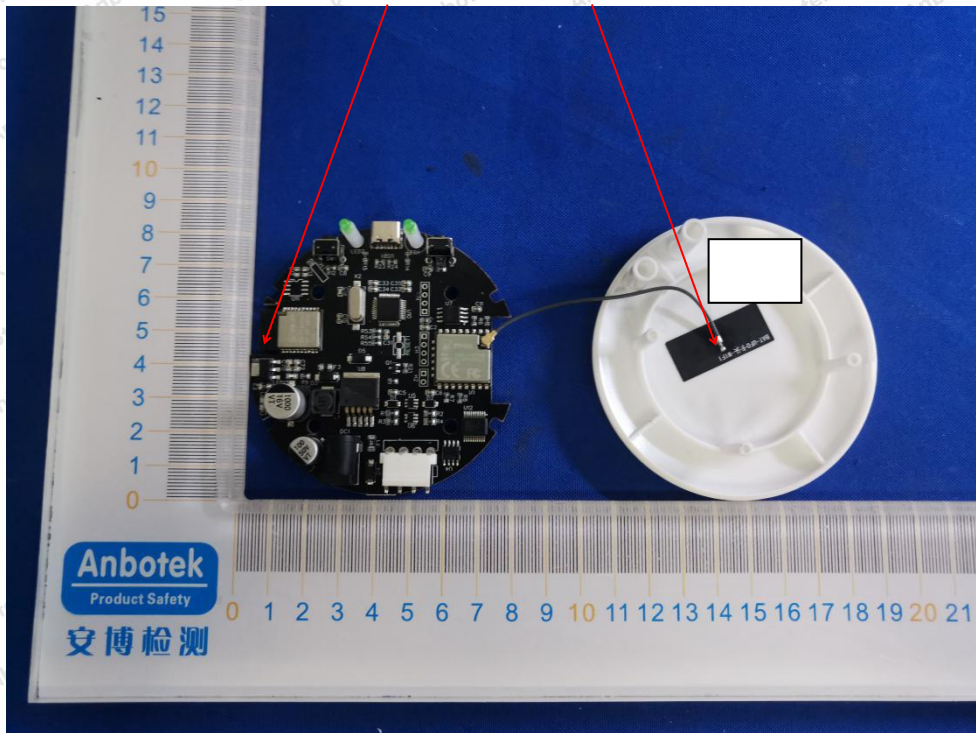
BLE ANT WIFI ANT
