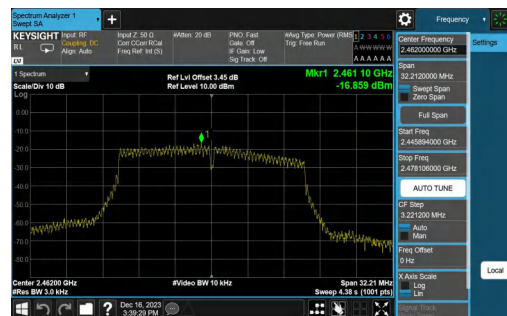
11G-CDD-Ant2-2462-PASS
