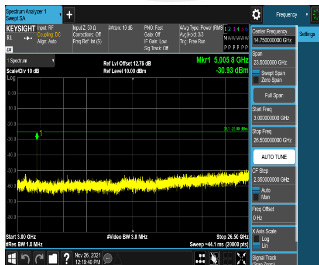
Band7-10MHz-16QAM-20800-50RB#0-Range3:3000~26500MHz
