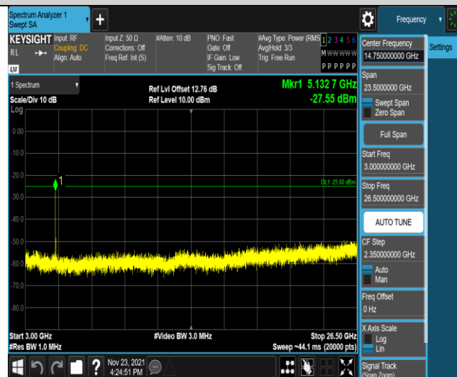
Band7-5MHz-QPSK-21425-25RB#0-Range3:3000~26500MHz
