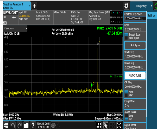
Band7-5MHz-QPSK-21425-25RB#0-Range2:1000~3000MHz
