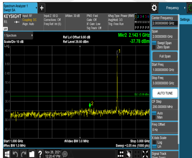
Band7-10MHz-16QAM-21400-50RB#0-Range2:1000~3000MHz
