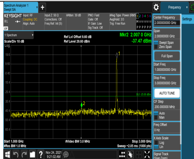
Band7-10MHz-QPSK-20800-50RB#0-Range2:1000~3000MHz
