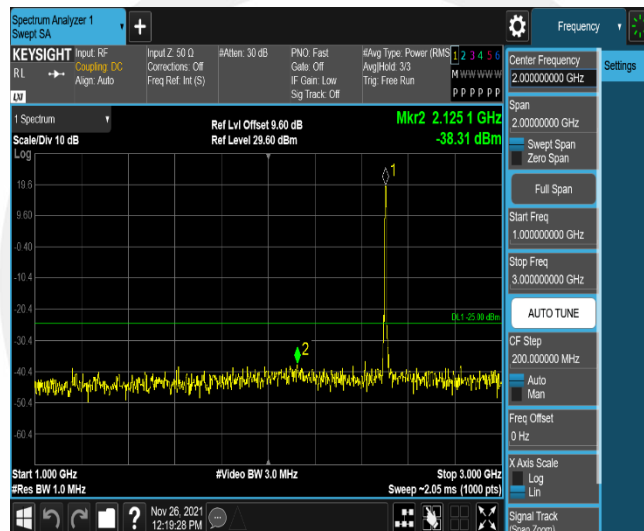
Band7-10MHz-16QAM-20800-50RB#0-Range2:1000~3000MHz
