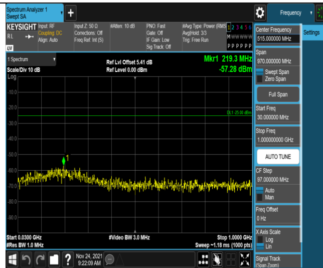
Band7-10MHz-QPSK-21100-50RB#0-Range1:30~1000MHz
