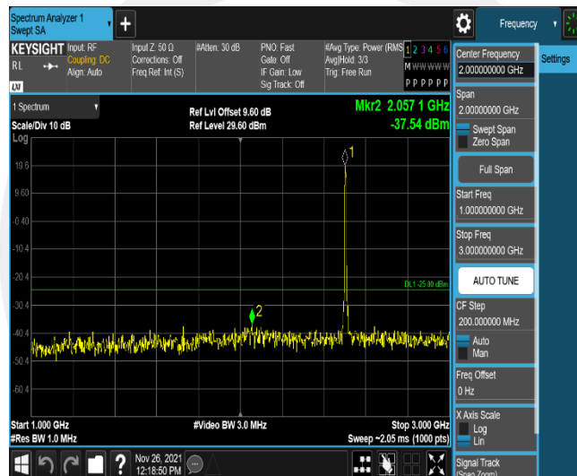
Band7-10MHz-16QAM-21100-50RB#0-Range2:1000~3000MHz
