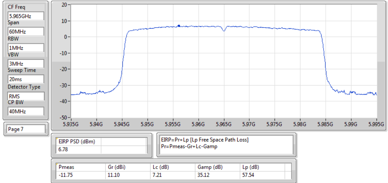
EIRP PSD;Band:6.2G;ax40,BF;BWch:40MHz;Nss:1,(M0);Nant:2;Ch:5965MHz;TX
