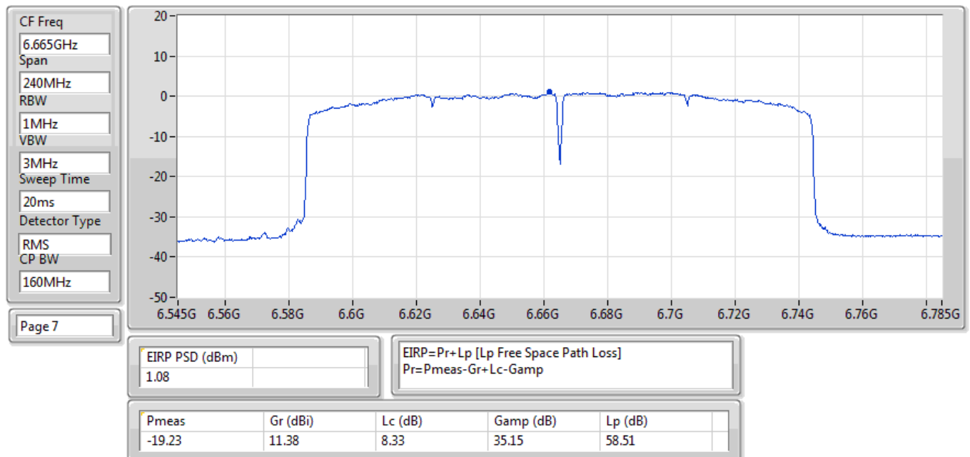
EIRP PSD;Band:6.7G;ax160,BF;BWch:160MHz;Nss:1,(M0);Nant:2;Ch:6665MHz;TX
