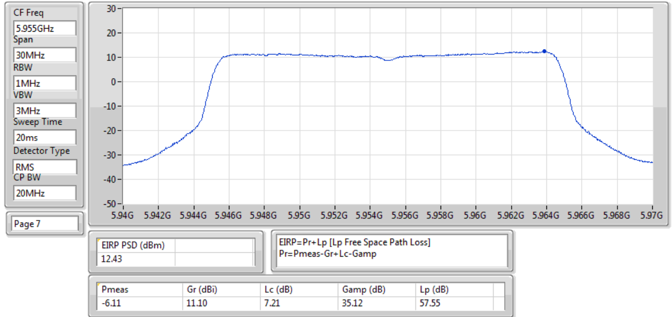
EIRP PSD;Band:6.2G;ax20,BF;BWch:20MHz;Nss:1,(M0);Nant:2;Ch:5955MHz;TX
