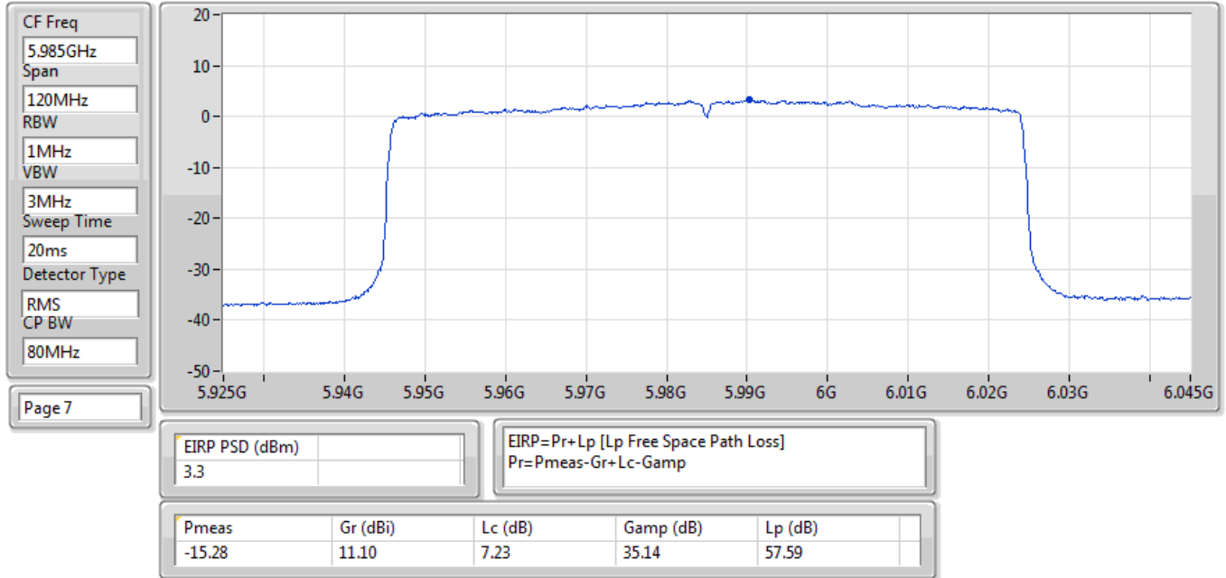
EIRP PSD;Band:6.2G;ax80,BF;BWch:80MHz;Nss:1,(M0);Nant:2;Ch:5985MHz;TX
