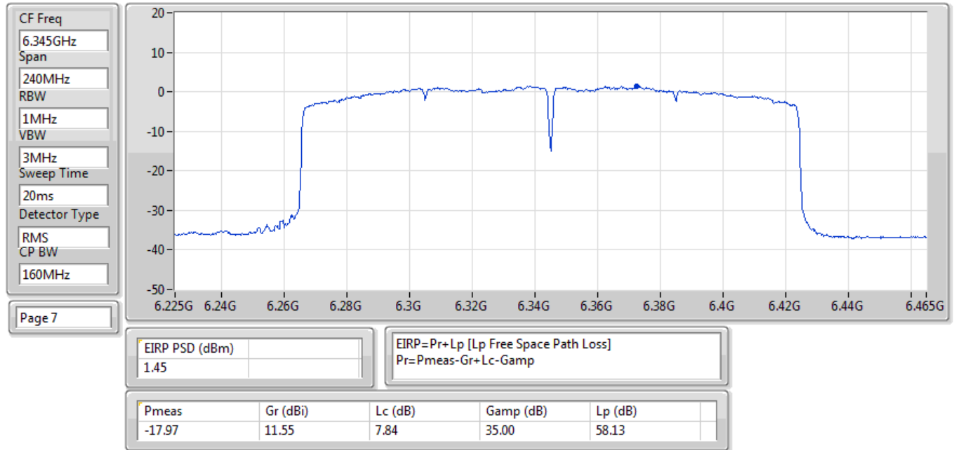
EIRP PSD;Band:6.2G;ax160,BF;BWch:160MHz;Nss:1,(M0);Nant:2;Ch:6345MHz;TX
