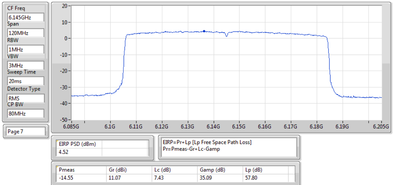
EIRP PSD;Band:6.2G;ax80,BF;BWch:80MHz;Nss:1,(M0);Nant:2;Ch:6145MHz;TX
