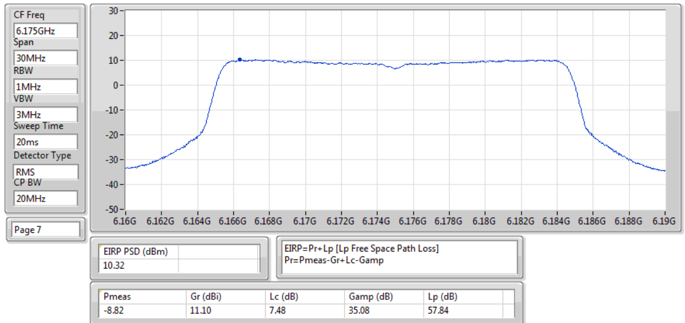
EIRP PSD;Band:6.2G;ax20,BF;BWch:20MHz;Nss:1,(M0);Nant:2;Ch:6175MHz;TX
