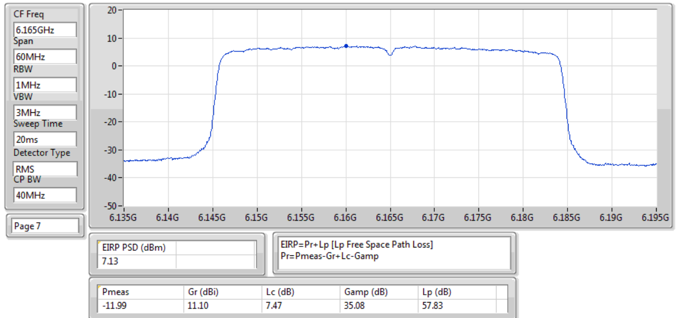
EIRP PSD;Band:6.2G;ax40,BF;BWch:40MHz;Nss:1,(M0);Nant:2;Ch:6165MHz;TX
