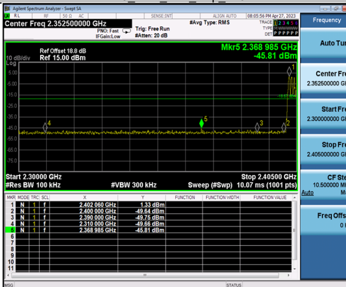
DH5_Ant1_Low_Hop_2402
