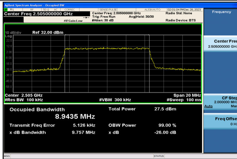
Band7-10MHz-QPSK-20800-50RB#0-8.9435
