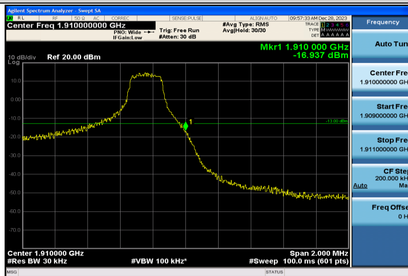
Band2-3MHz-QPSK-19185-1RB#14
