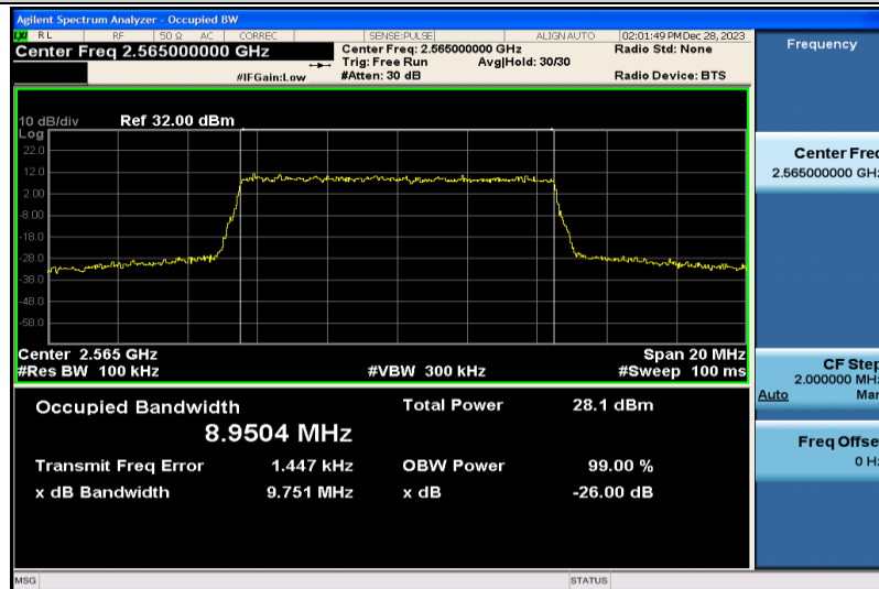
Band7-10MHz-QPSK-21400-50RB#0-8.9504
