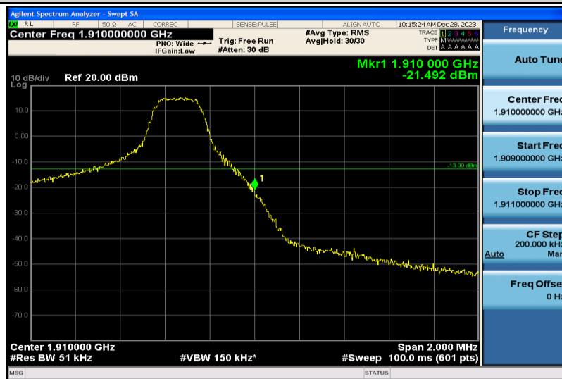
Band2-5MHz-QPSK-19175-1RB#24
