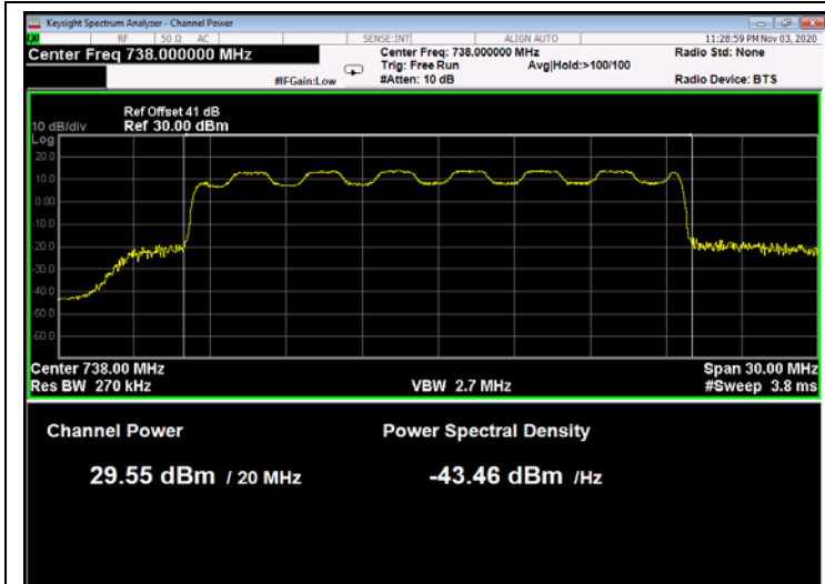
Figure 32: 16QAM 20MHz B.W.; 738.0MHz, 15kHz
