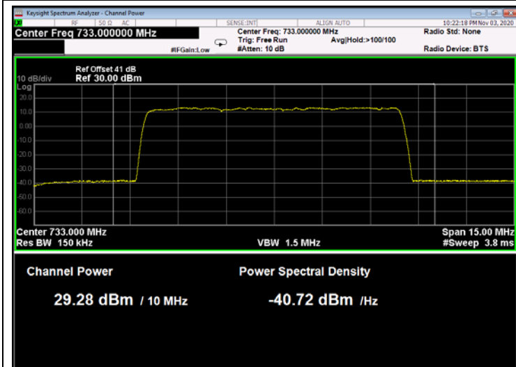
Figure 49: 64QAM 10MHz B.W.; 733.0MHz, 60kHz
