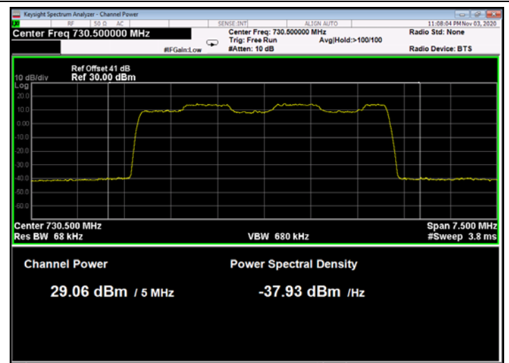
Figure 9: 16QAM 5MHz B.W.; 730.5MHz, 30kHz
