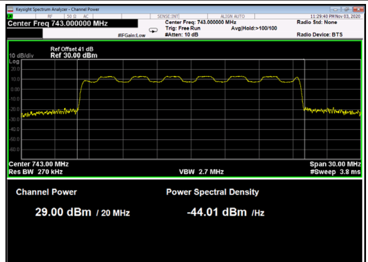
Figure 35: 16QAM 20MHz B.W.; 743.0MHz, 15kHz
