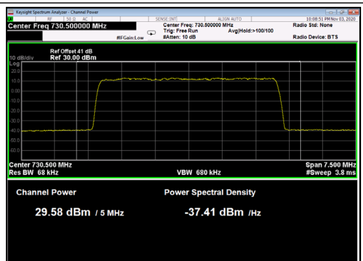
Figure 42: 64QAM 5MHz B.W.; 730.5MHz, 30kHz
