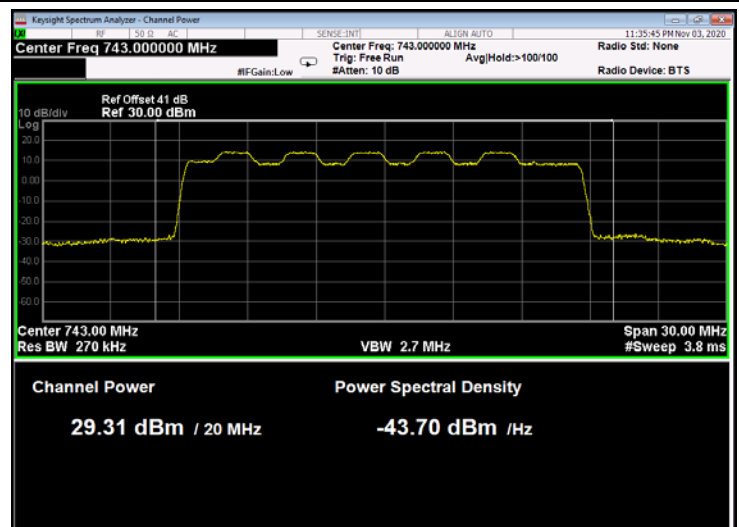
Figure 37: 16QAM 20MHz B.W.; 743.0MHz, 60kHz
