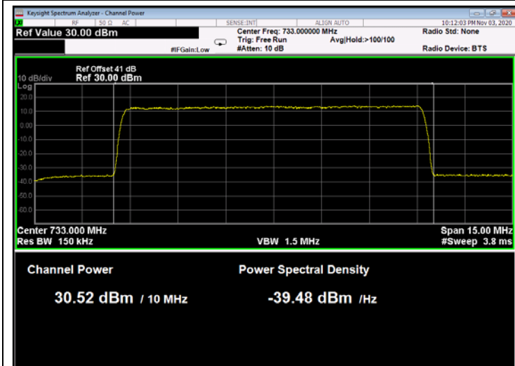
Figure 47: 64QAM 10MHz B.W.; 733.0MHz, 15kHz
