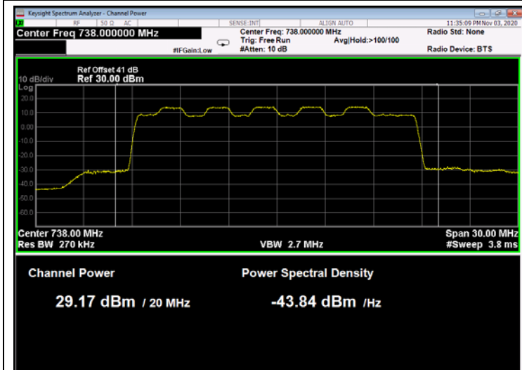
Figure 34: 16QAM 20MHz B.W.; 738.0MHz, 60kHz
