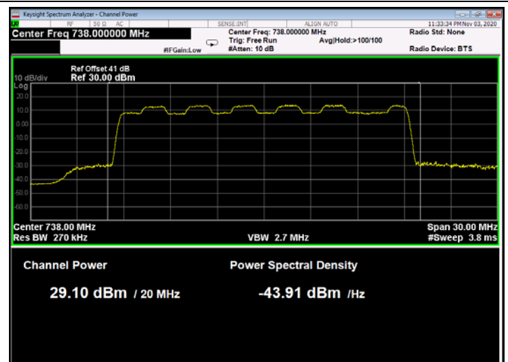
Figure 33: 16QAM 20MHz B.W.; 738.0MHz, 30kHz
