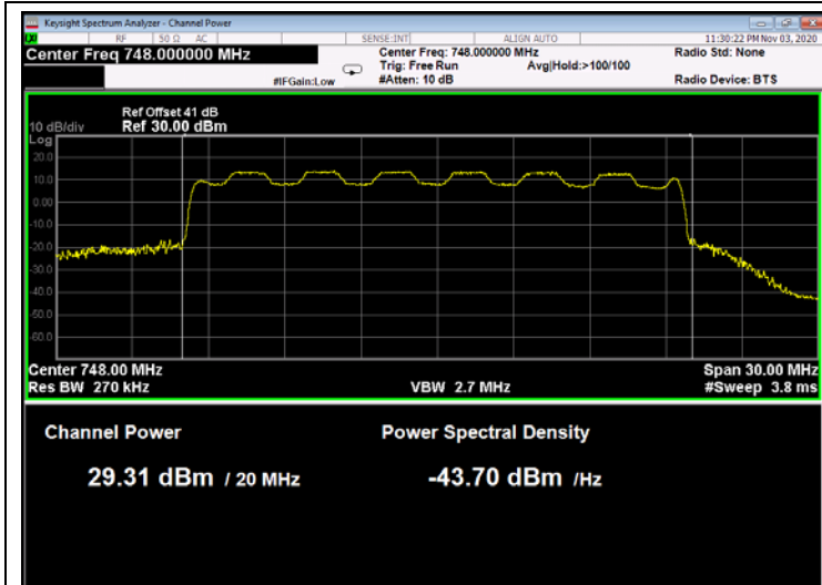
Figure 38: 16QAM 20MHz B.W.; 748.0MHz, 15kHz
