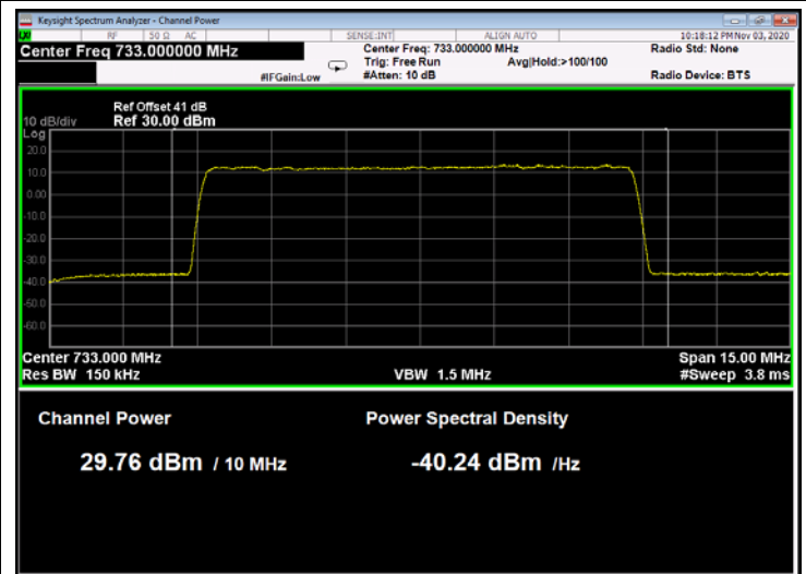
Figure 48: 64QAM 10MHz B.W.; 733.0MHz, 30kHz
