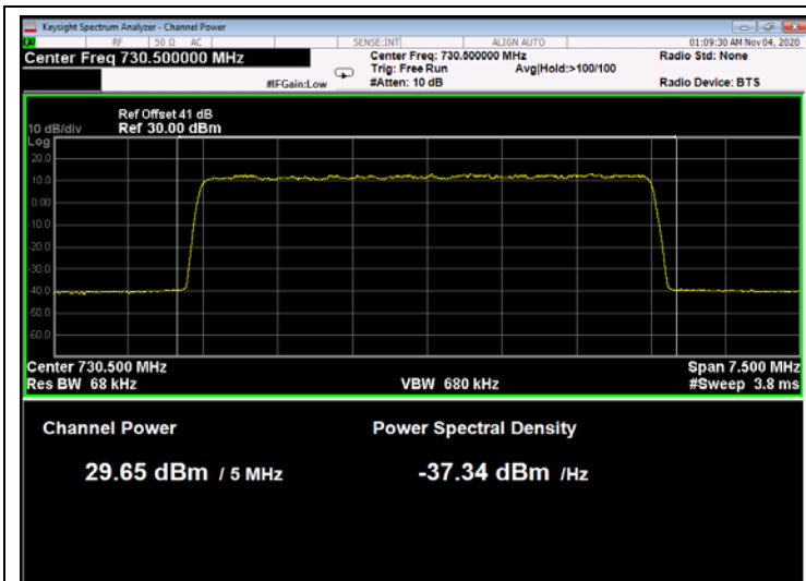
Figure 74: 256QAM 5MHz B.W.; 730.5.5MHz, 15kHz
