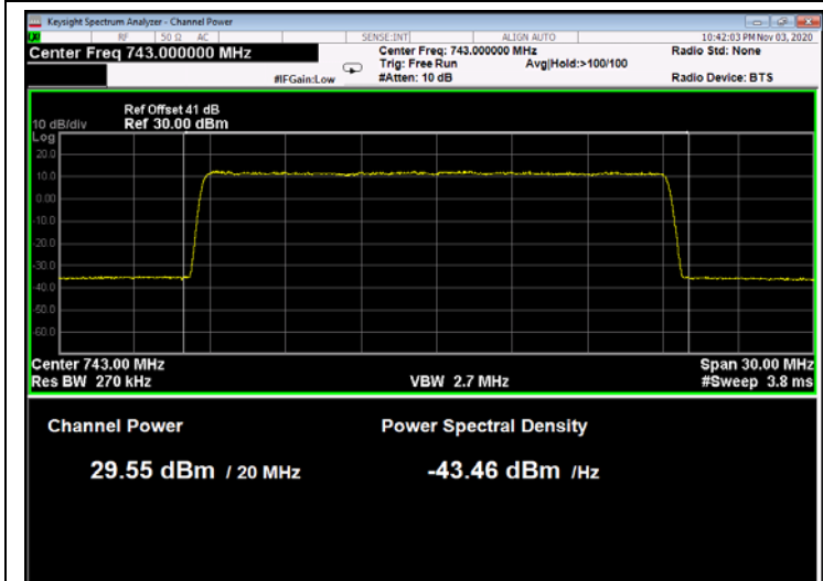
Figure 69: 64QAM 20MHz B.W.; 743.0MHz, 30kHz
