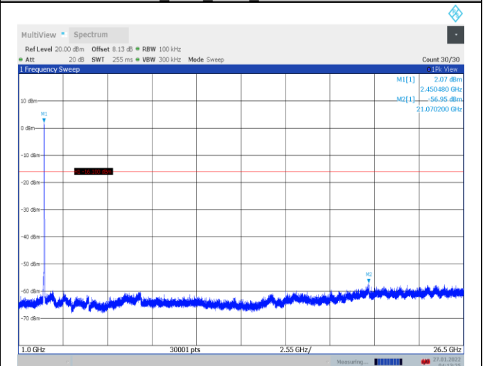
11G_Ant1_2457_1000~26500
