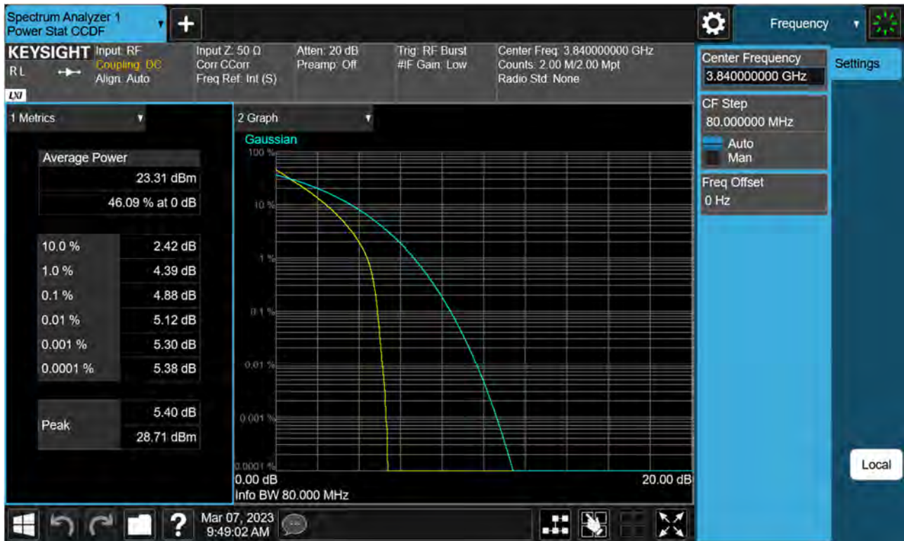
Sub6 n77(78). PAR Plot (80 M BW_Ch.656000_QPSK)
