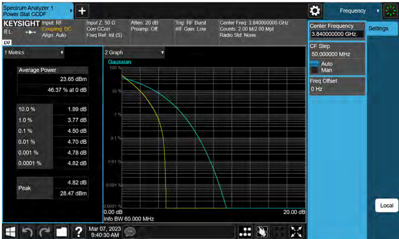
Sub6 n77(78). PAR Plot (60 M BW_Ch.656000_BPSK)
