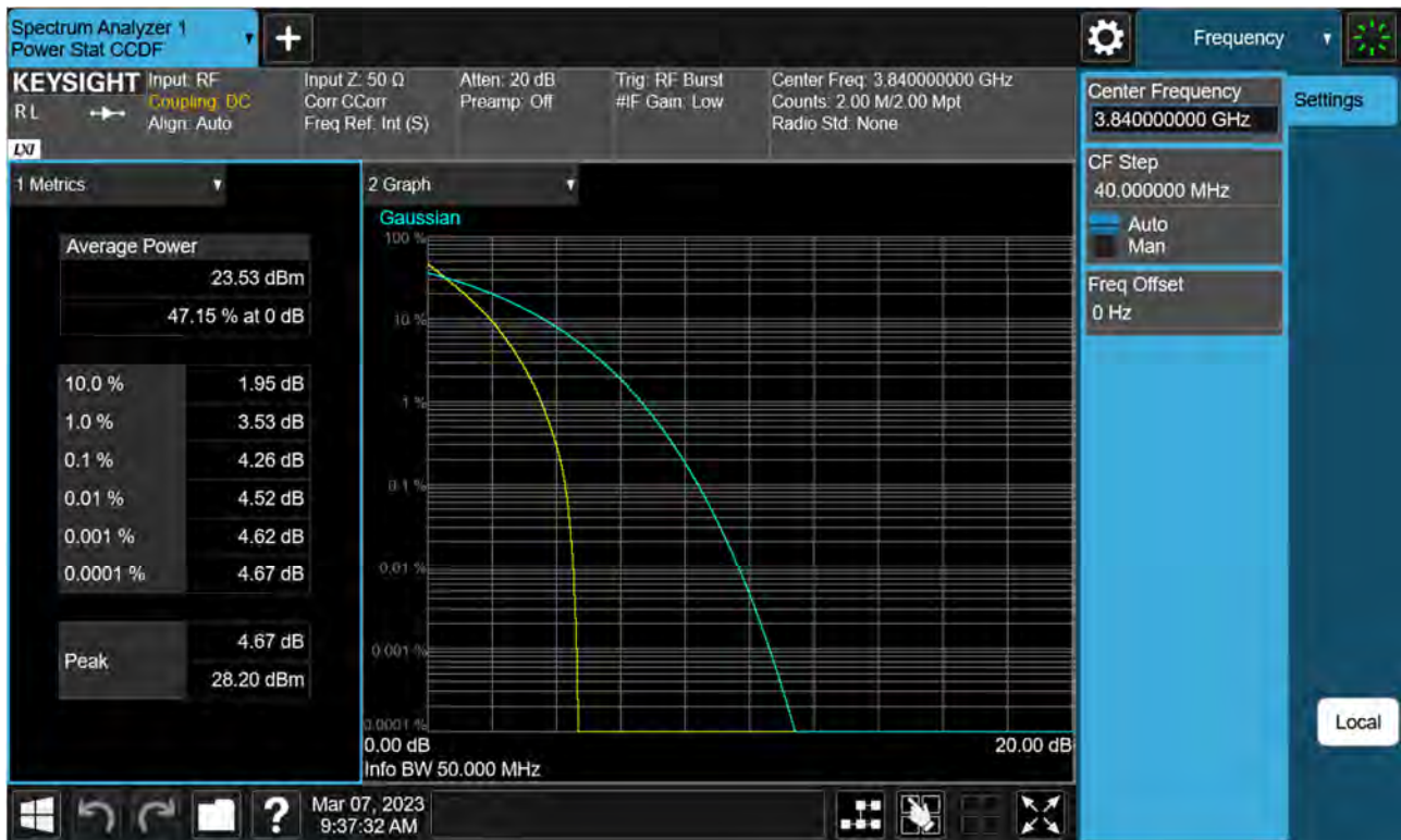
Sub6 n77(78). PAR Plot (50 M BW_Ch.656000_BPSK)
