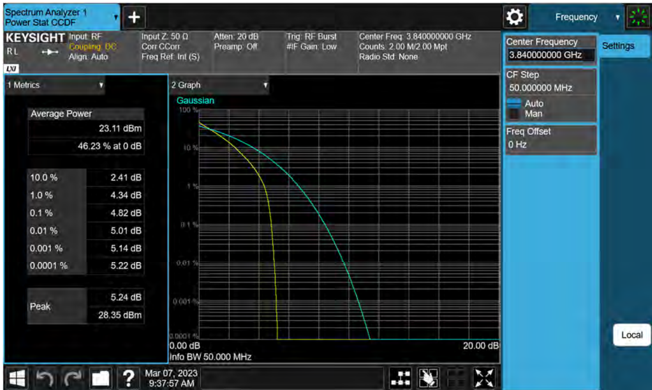
Sub6 n77(78). PAR Plot (50 M BW_Ch.656000_QPSK)
