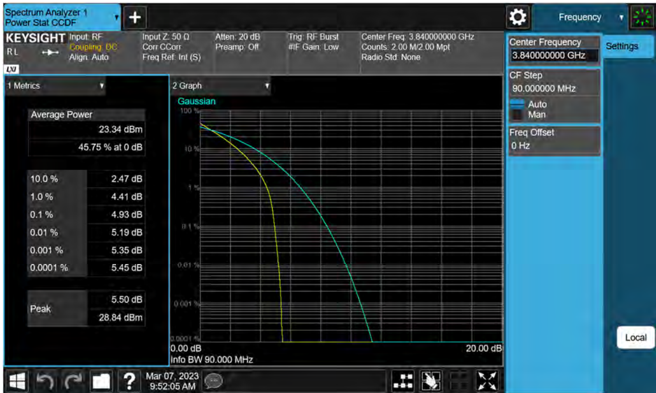
Sub6 n77(78). PAR Plot (90 M BW_Ch.656000_QPSK)
