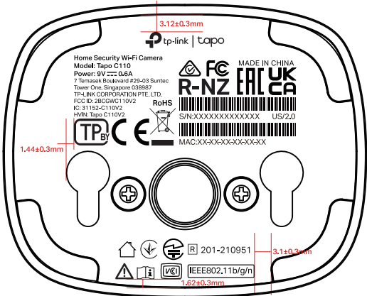
尺寸图
