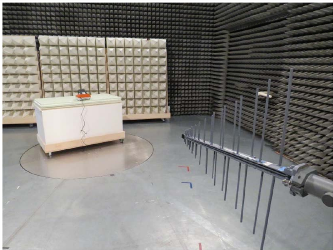
EUT CONFIGURATION I - HL 223
