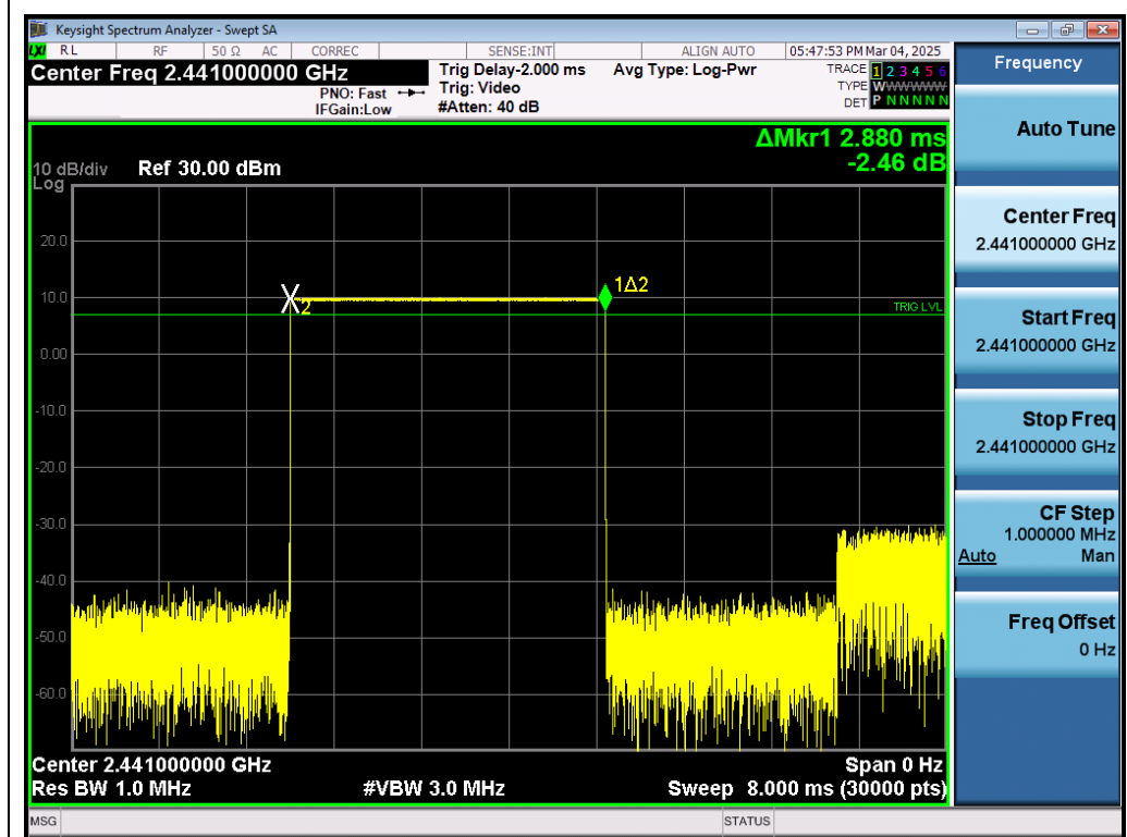
Test_Graph_BR_HOP_ANT1_NA_1Mbps_2441_Time per Burst
