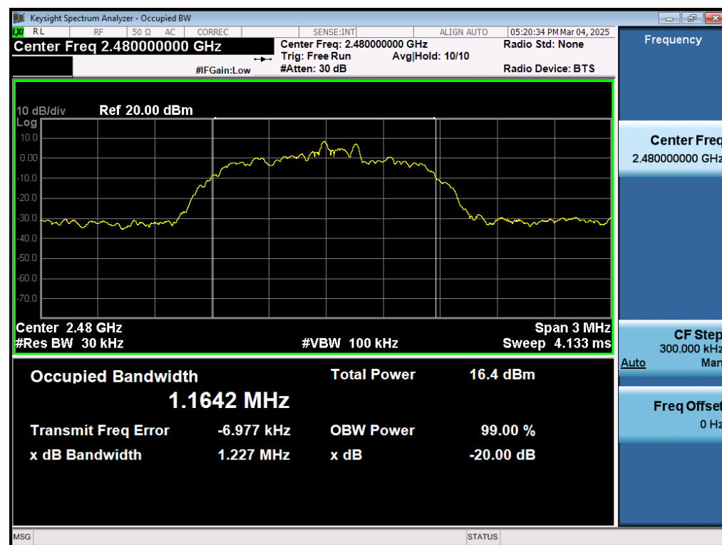
Test_Graph_EDR_ANT1_2480_2Mbps_OBW
