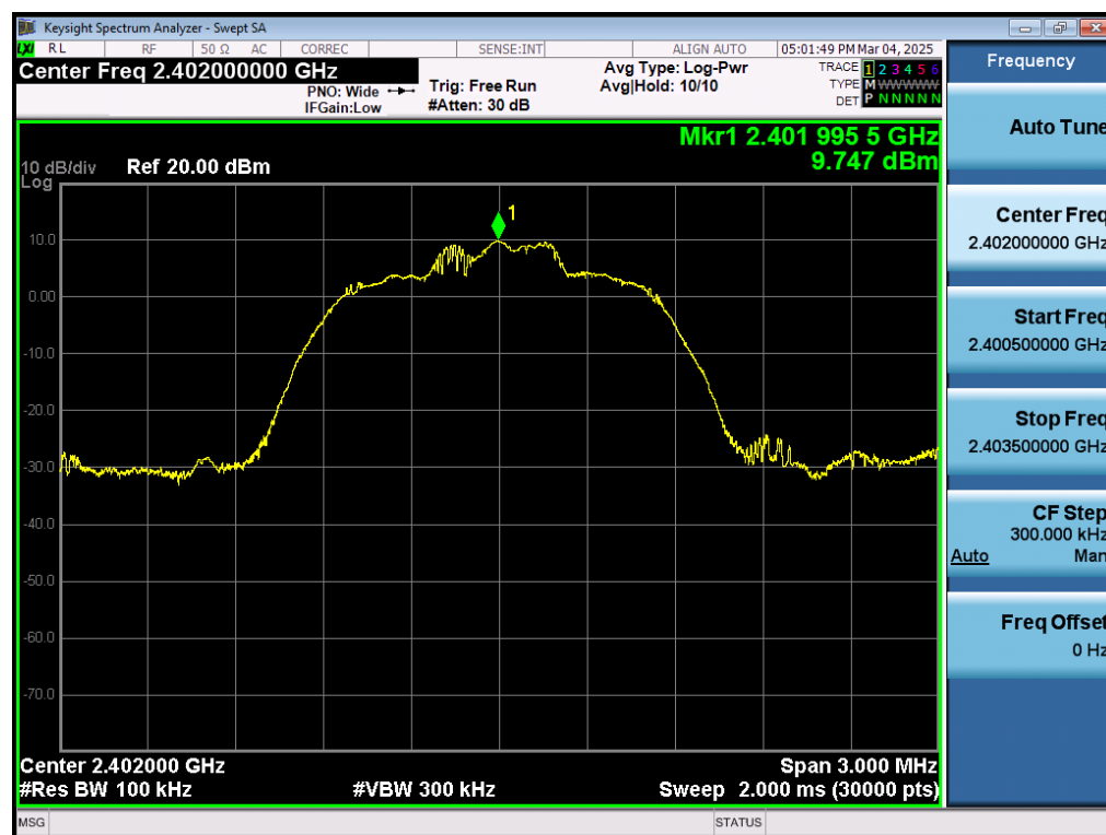
Test_Graph_EDR_ANT1_2402_2Mbps_Reference Level
