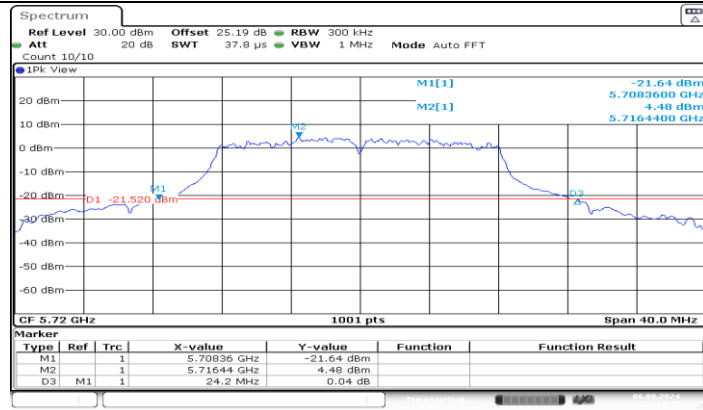
11A_Ant1_5720
