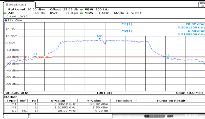
11N20MIMO_Ant1_5320
