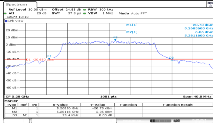
11N20MIMO_Ant1_5280
