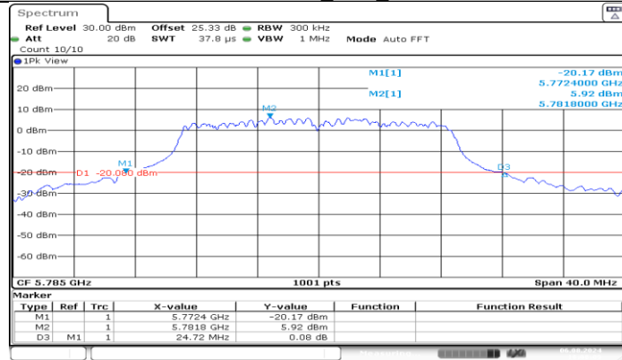
11N20MIMO_Ant1_5785
