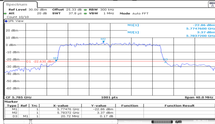
11AX20MIMO_Ant1_5785
