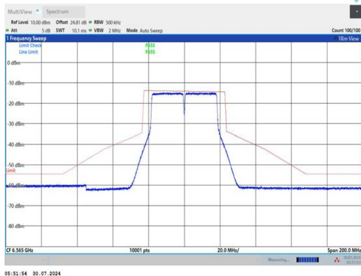
11AC40MIMO_Ant2_6565
