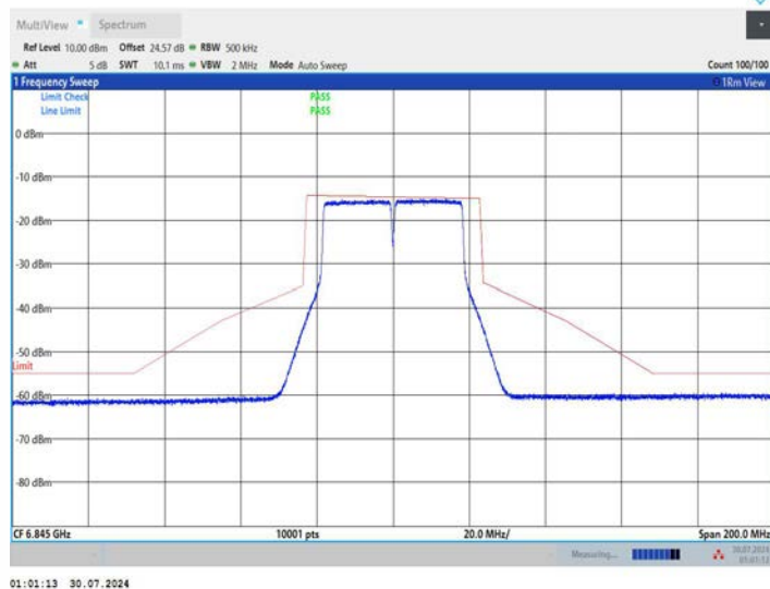
11N40MIMO_Ant2_6845
