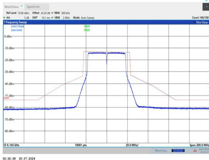
11AC40MIMO_Ant2_6165
