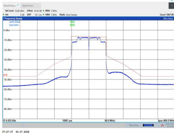
11AC160MIMO_Ant2_6025
