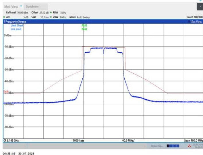
11AC80MIMO_Ant2_6145
