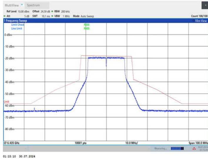
11AC20MIMO_Ant2_6435
