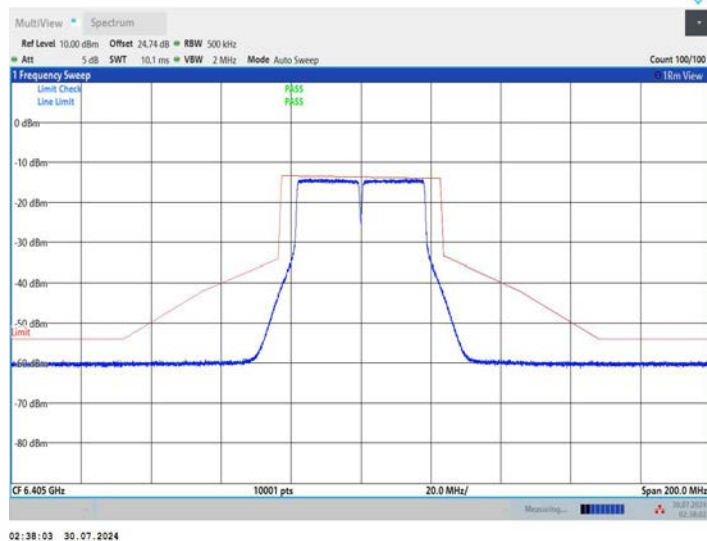
11AC40MIMO_Ant2_6405
