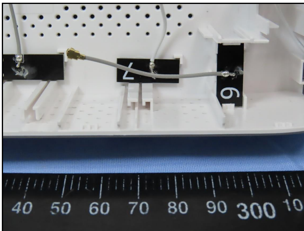
5G_ANT6
