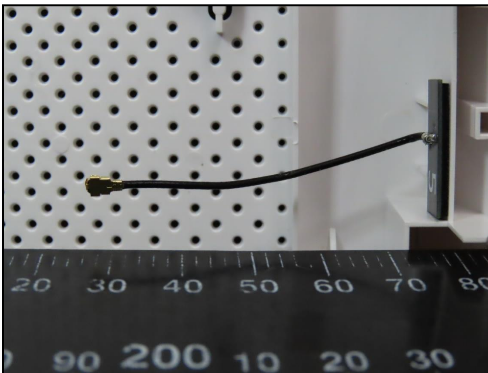
5G_ANT5
