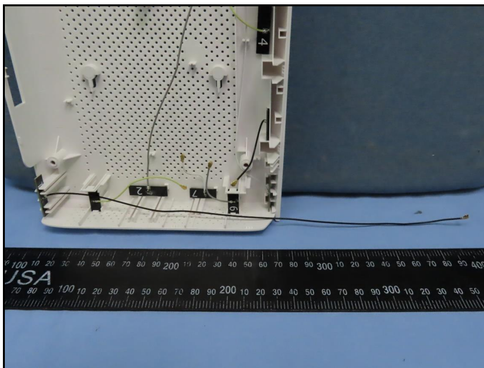
2G_ANT1
