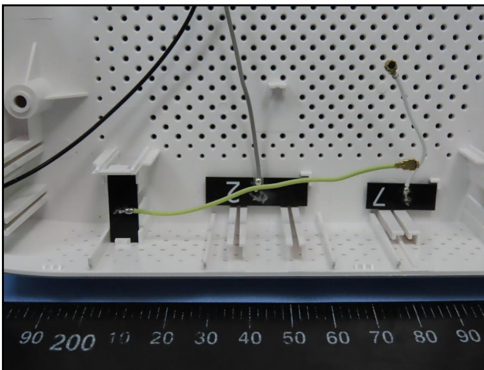
5G_ANT8
